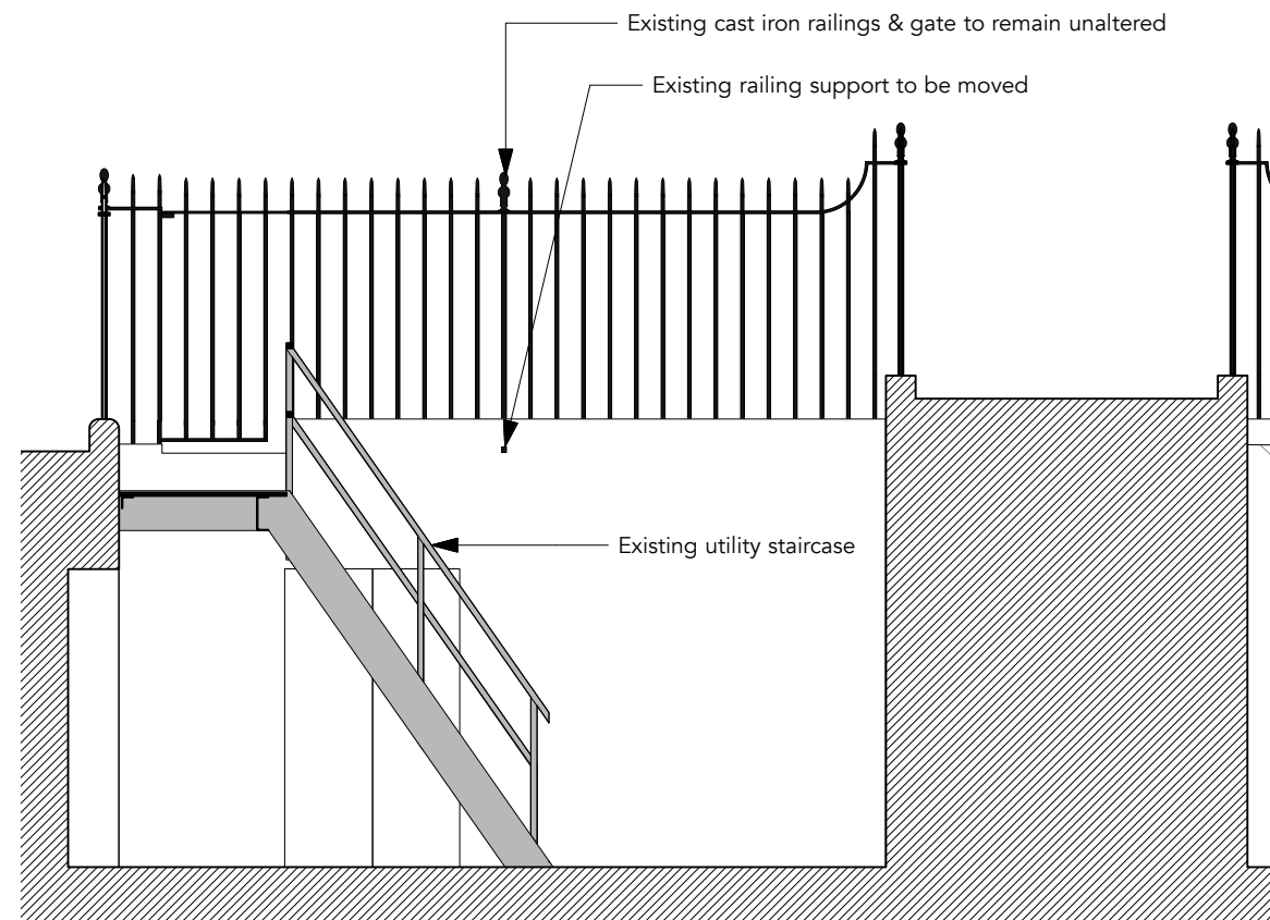
4 Existing Section A-A 1:50
