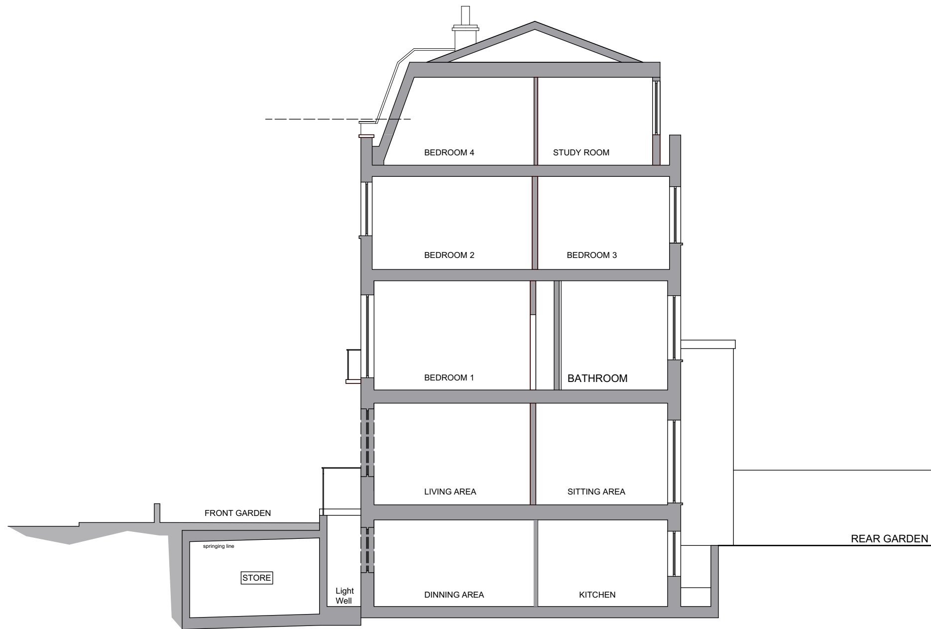
SECTION A-A
