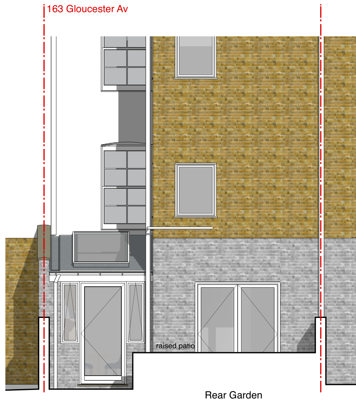
Section DD
