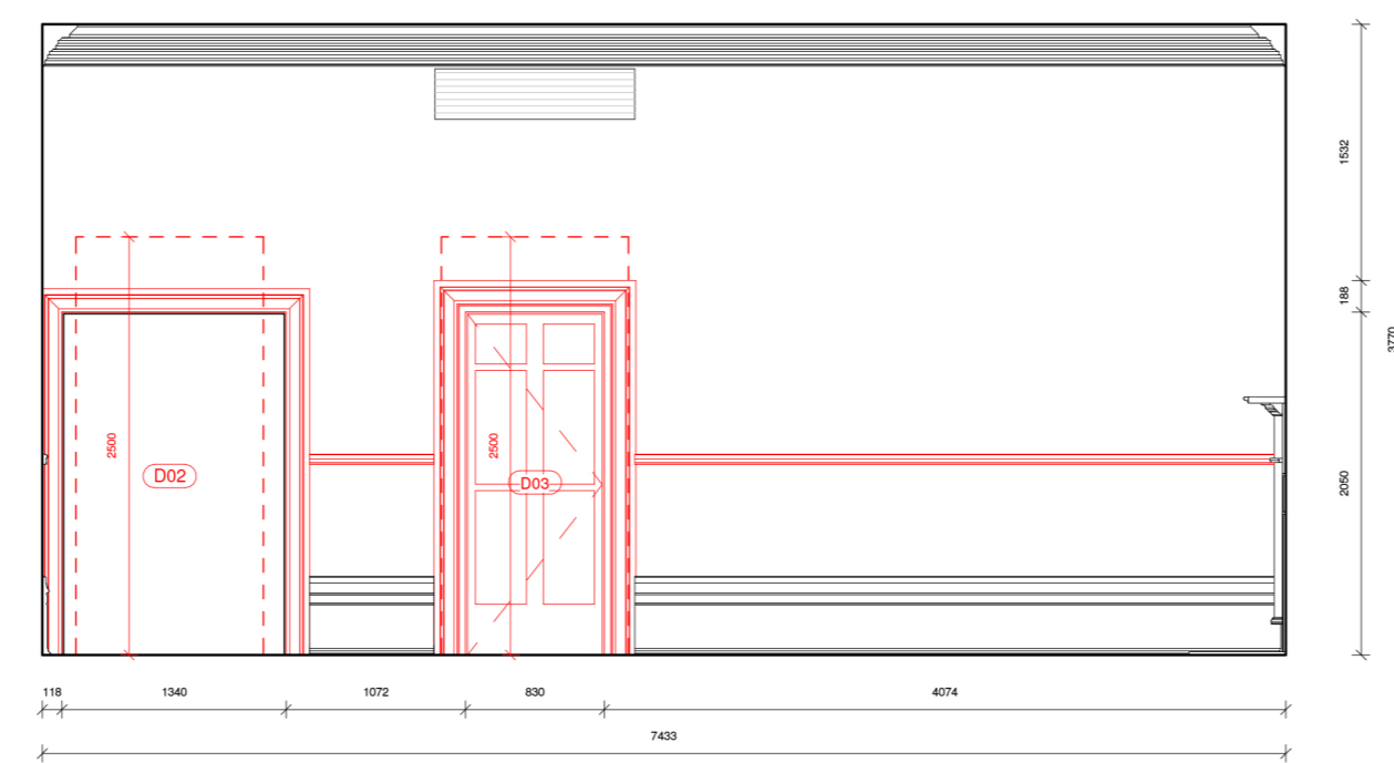
8 Elevation 4 - Demo 1 : 50
