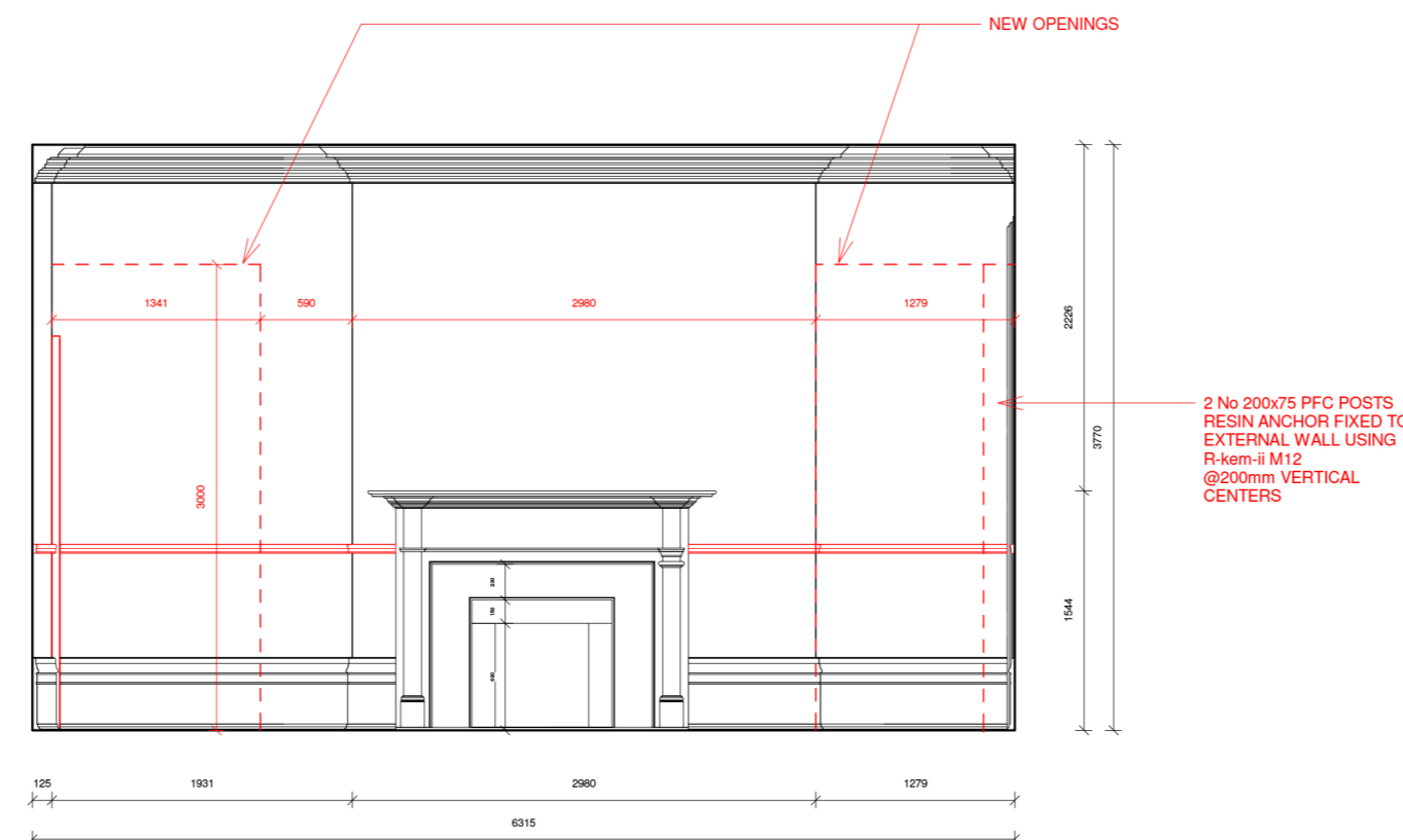
6 Elevation 2 - Demo 1 : 50
