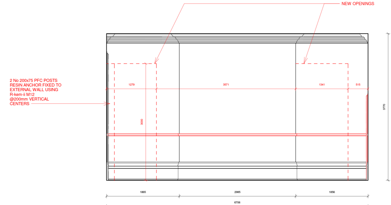
7 Elevation 3 - Demo 1 : 50
