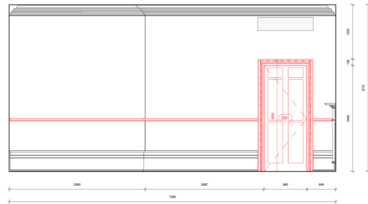
5 Elevation 1 - Demo 1 : 50
