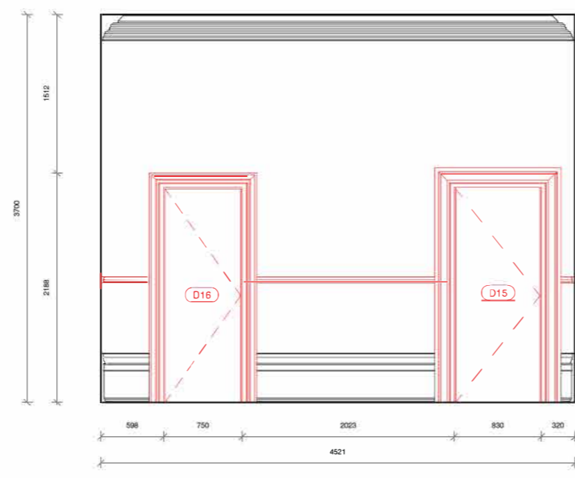
41 Elevation 19 - Demo 1 : 50
