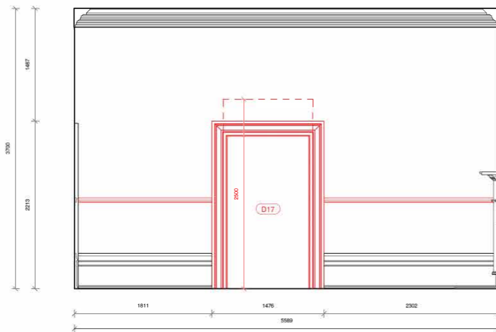
42 Elevation 20 - Demo 1 : 50
