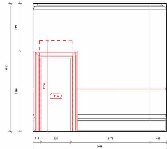
34 Elevation 15 - Demo 1 : 50
