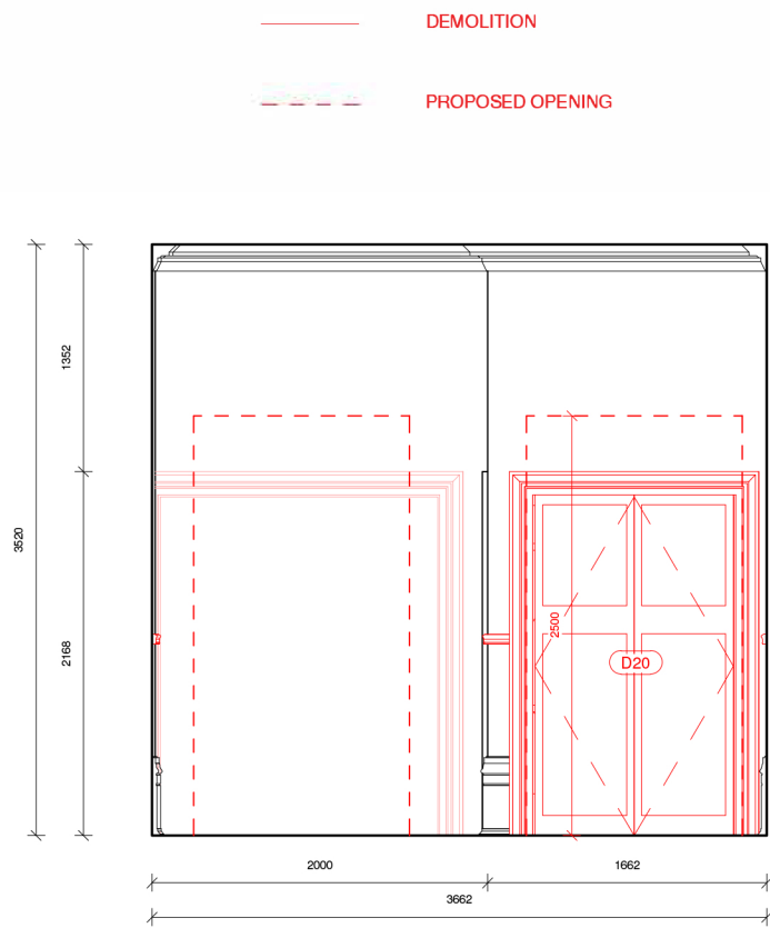
33 Elevation 14 - Demo 1 : 50
