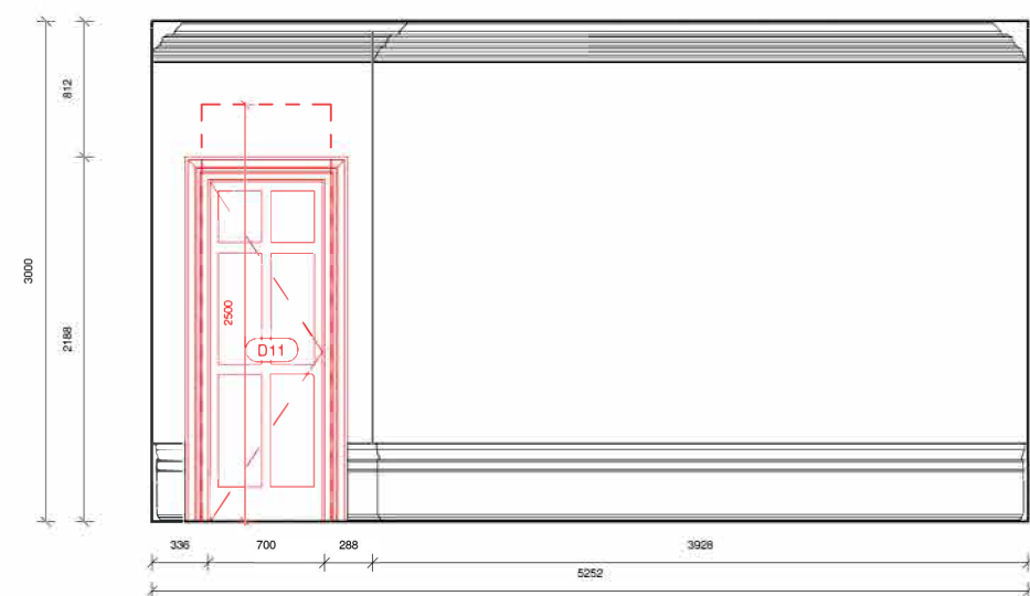
36 Elevation 17 - Demo 1 : 50
