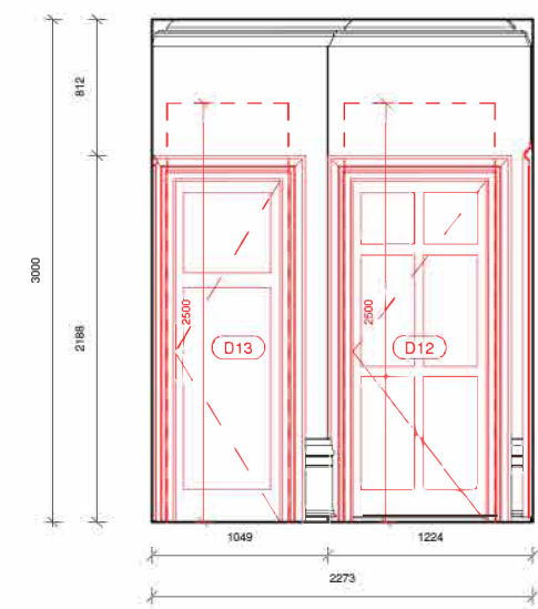
35 Elevation 16 - Demo 1 : 50
