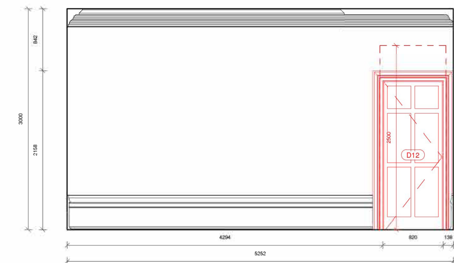
37 Elevation 18 - Demo 1 : 50
