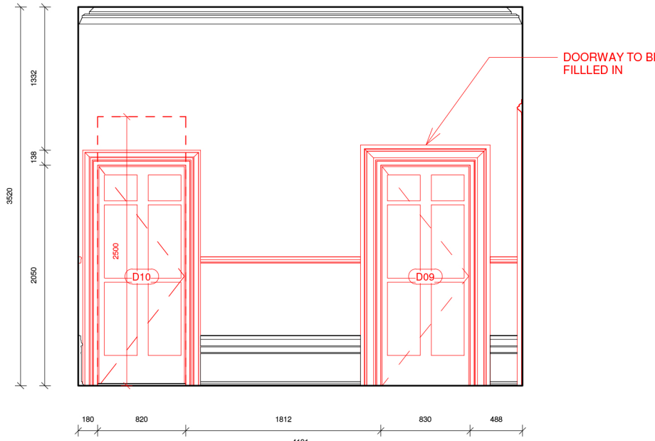
26 Elevation 12 - Demo 1 : 50
