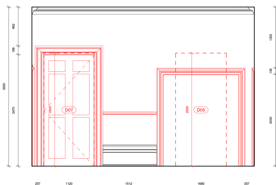
27 Elevation 13 - Demo 1 : 50
