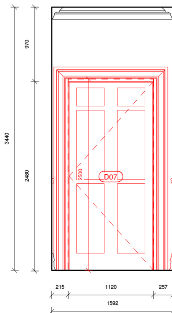
22 Elevation 9 - Demo 1 : 50
