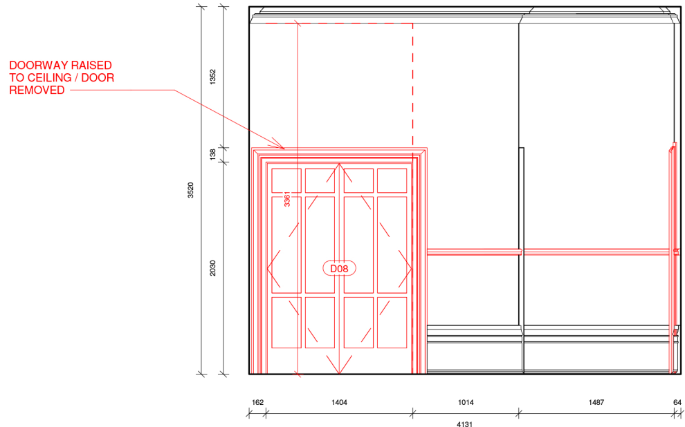
25 Elevation 11 - Demo 1 : 50
