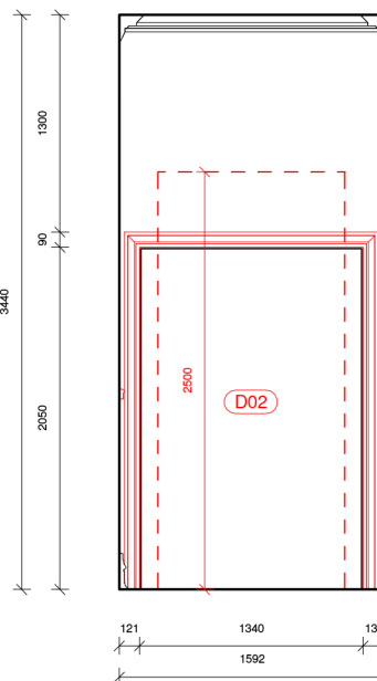
24 Elevation 10 - Demo 1 : 50
