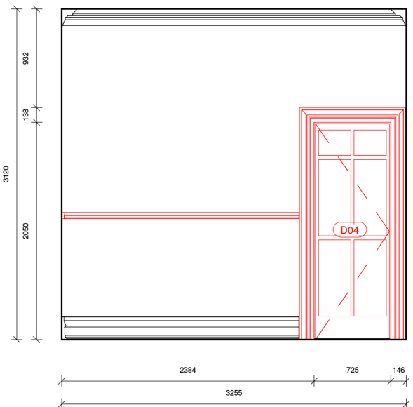
13 Elevation 5 - Demo 1 : 50
