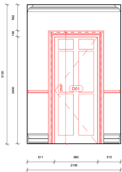
15 Elevation 7 - Demo 1 : 50
