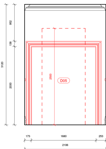
14 Elevation 6 - Demo 1 : 50
