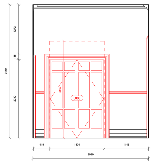
16 Elevation 8 - Demo 1 : 50
