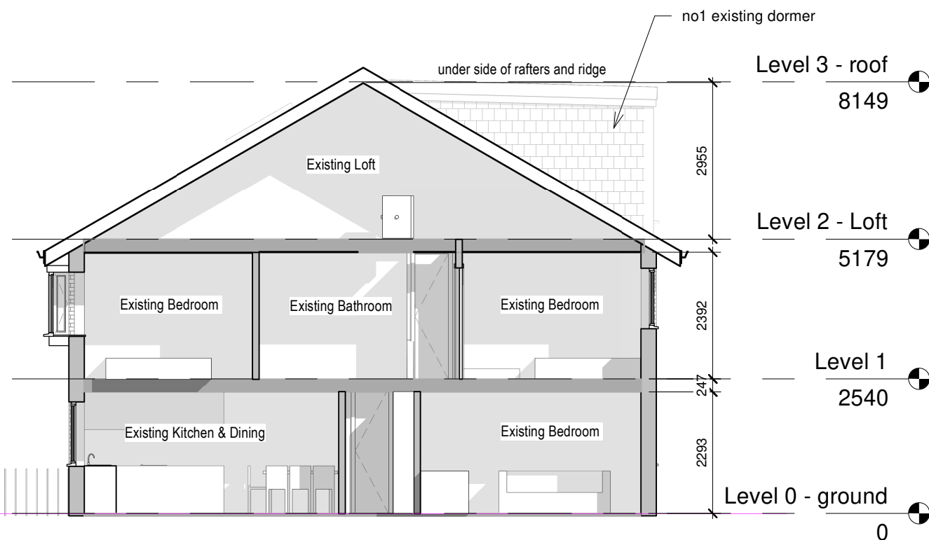
1 A300 Section 1 - existing 1 : 100
