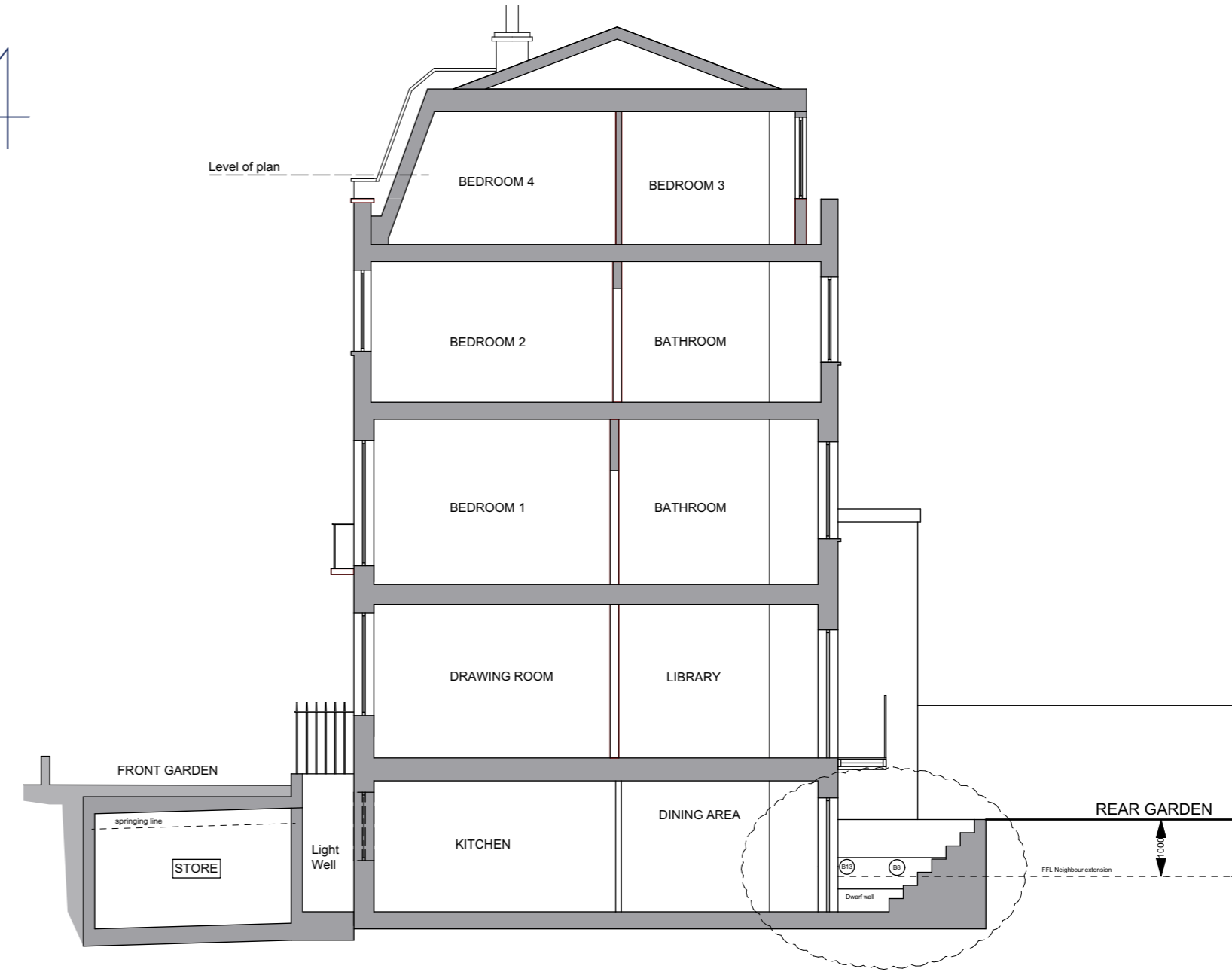
SECTION A-A
