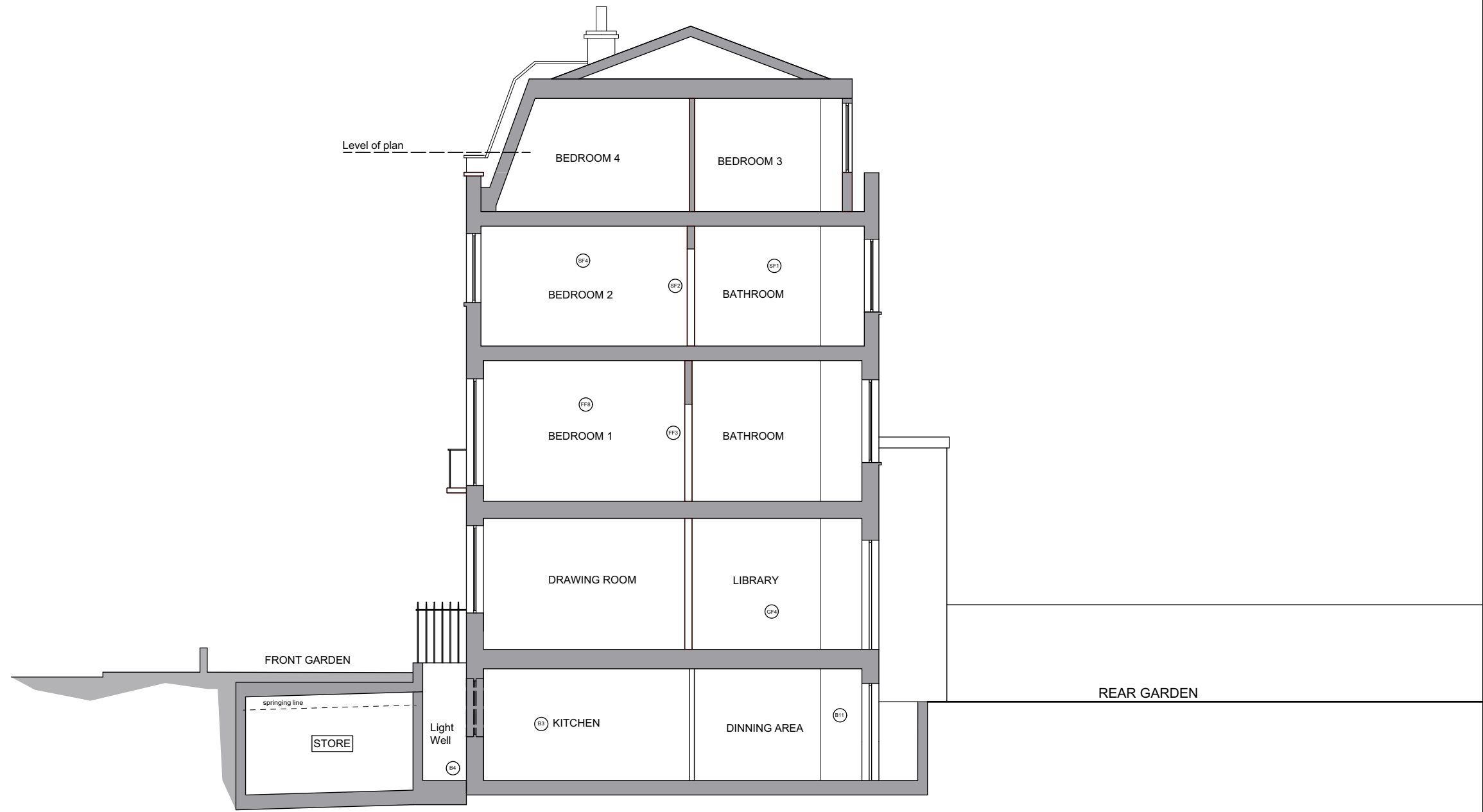
SECTION A-A
