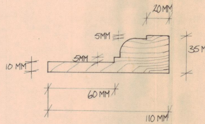
ARCHITRAVE 1:2
