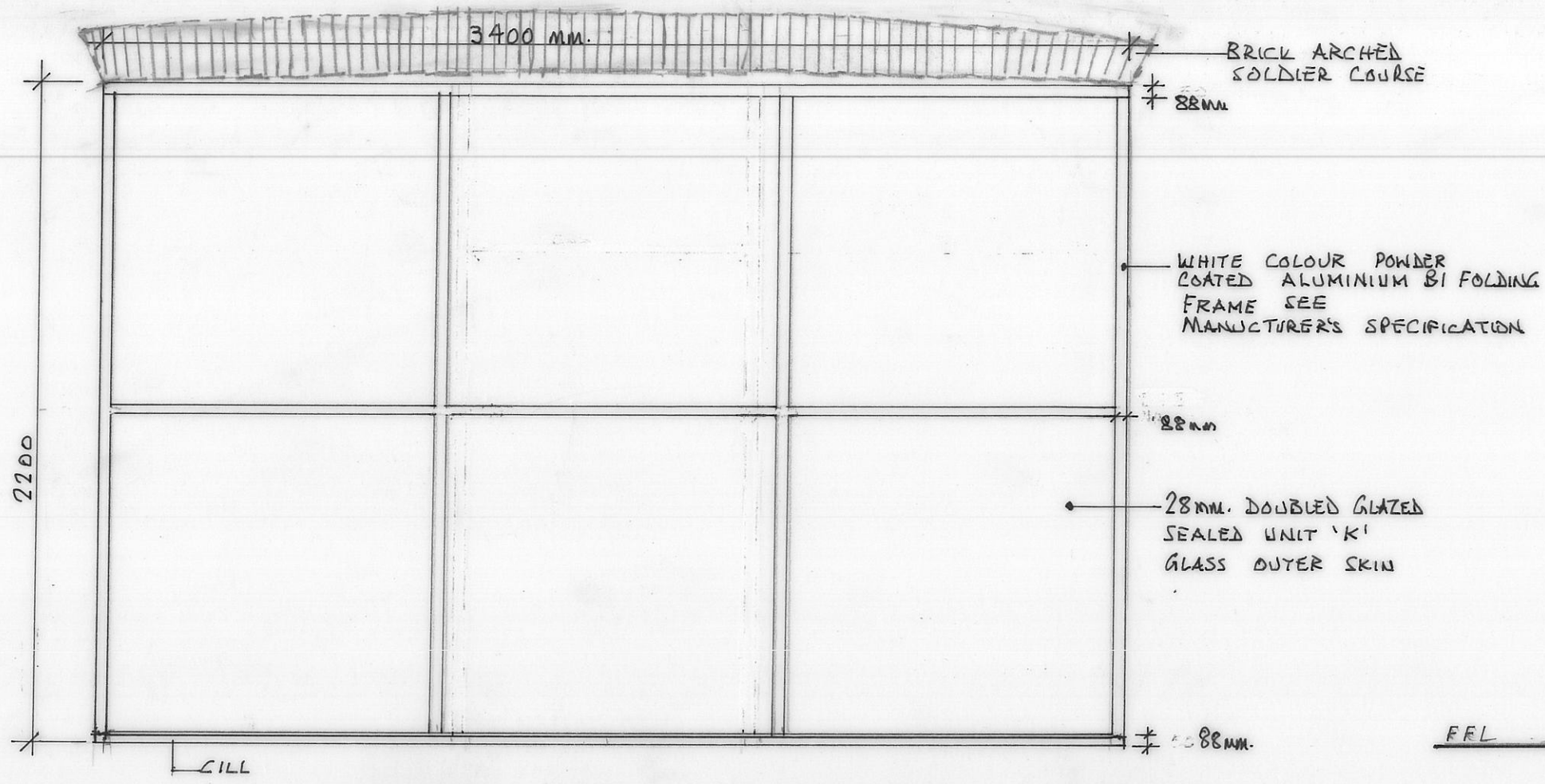
FLANK ELEVATION
