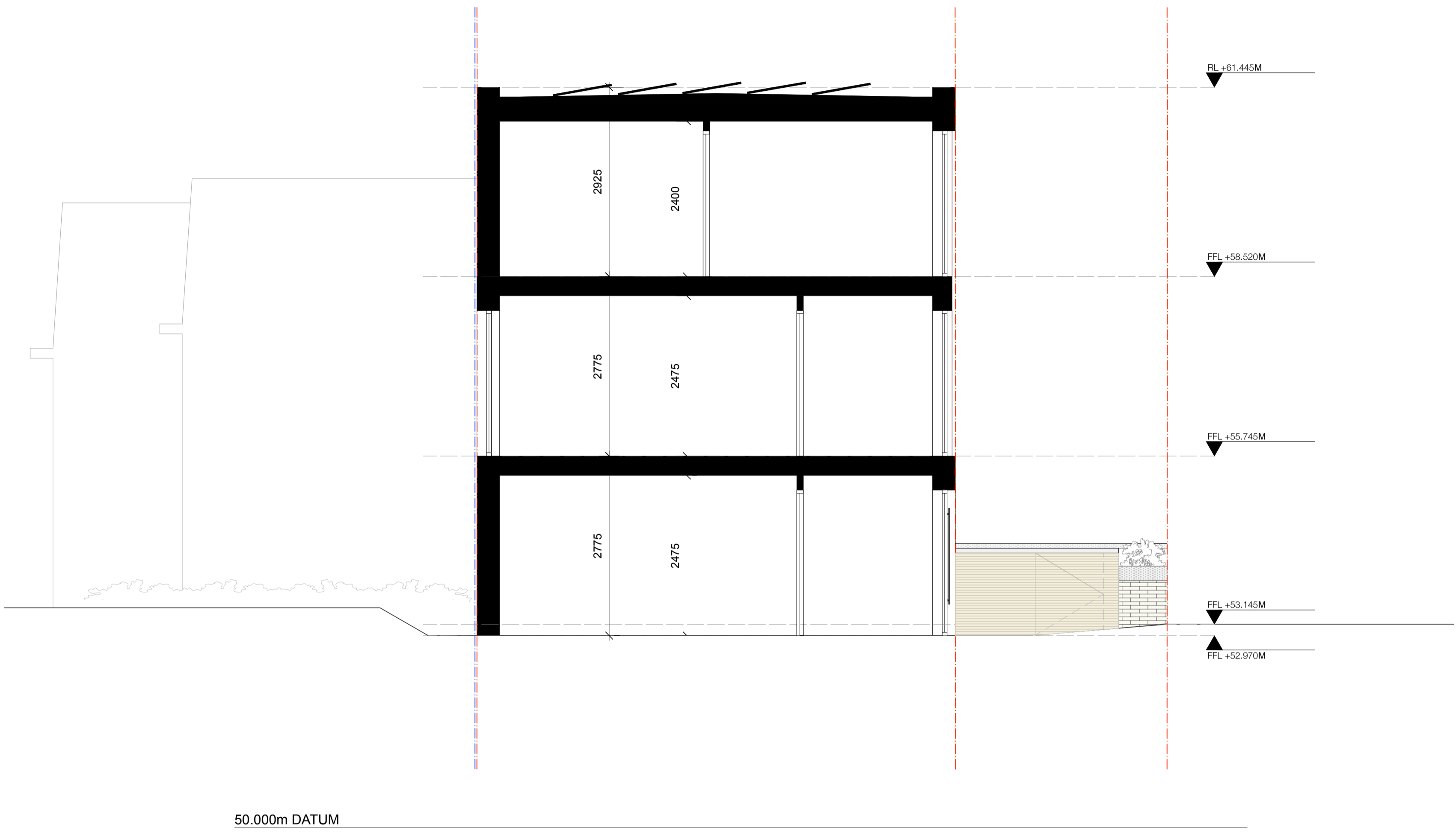
SECTION AA SCALE 1:50 @ A1 / 1:100 @ A3
