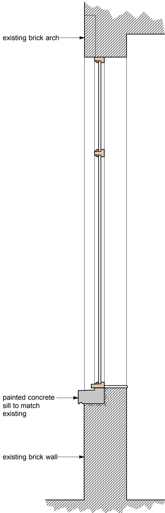
Section 1:20 @ A3
