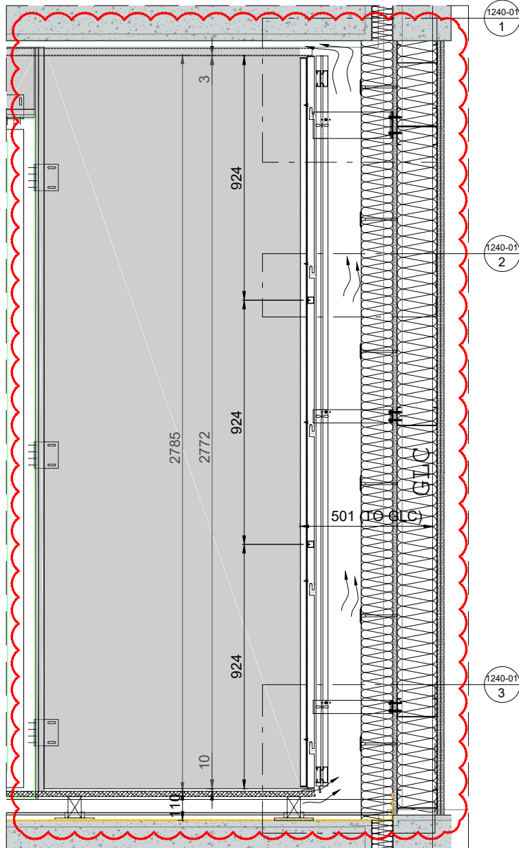
SECTION A-A
