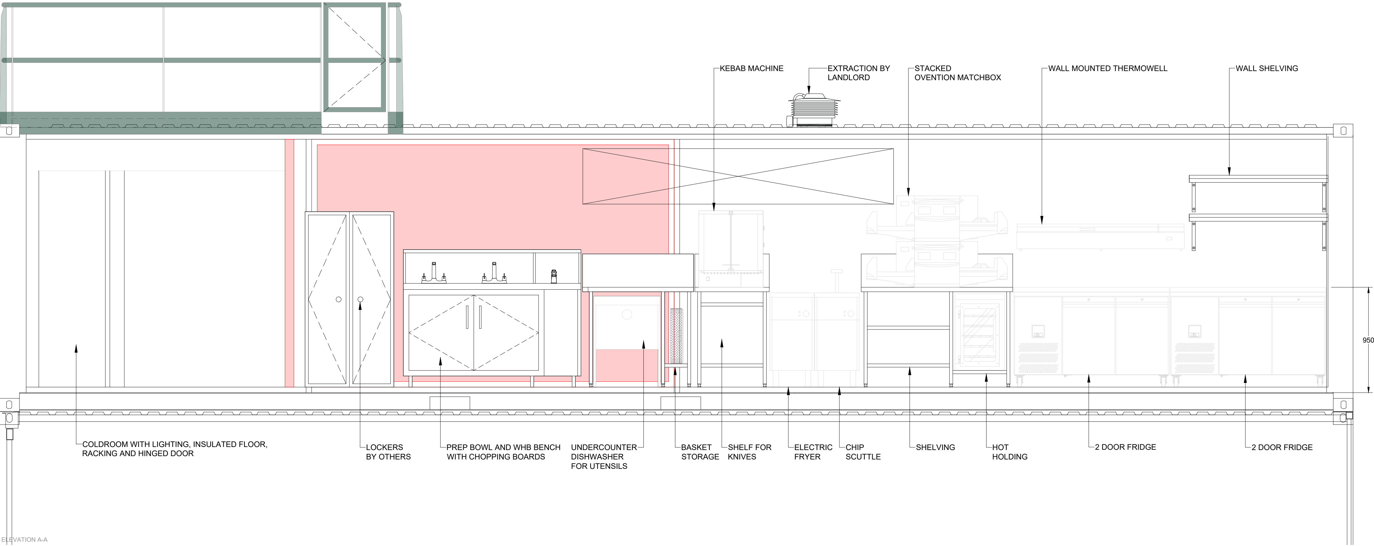
01 ELEVATION A-A SCALE 1:50 @ A1
