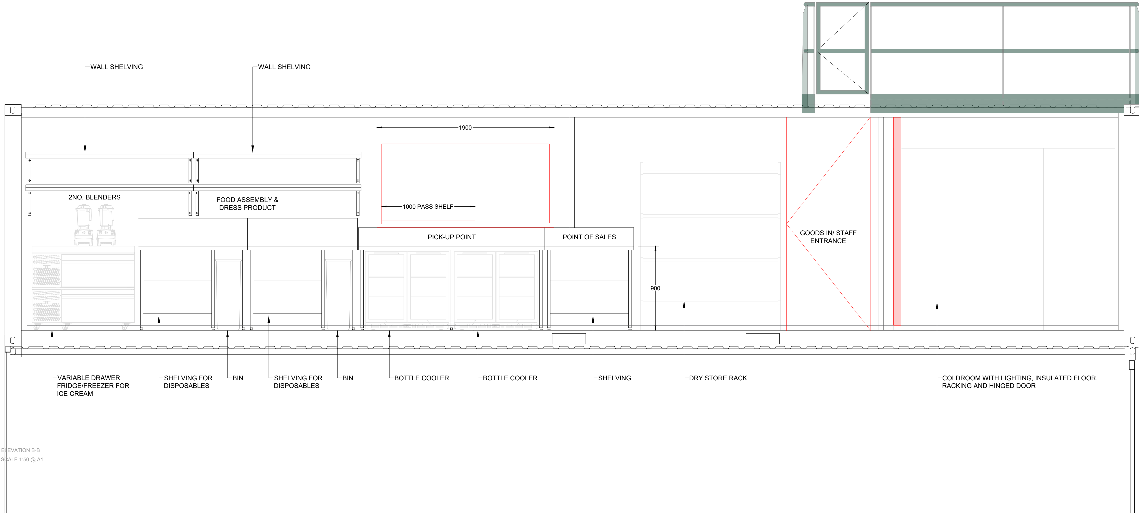
01 ELEVATION A-A SCALE 1:50 @ A1
