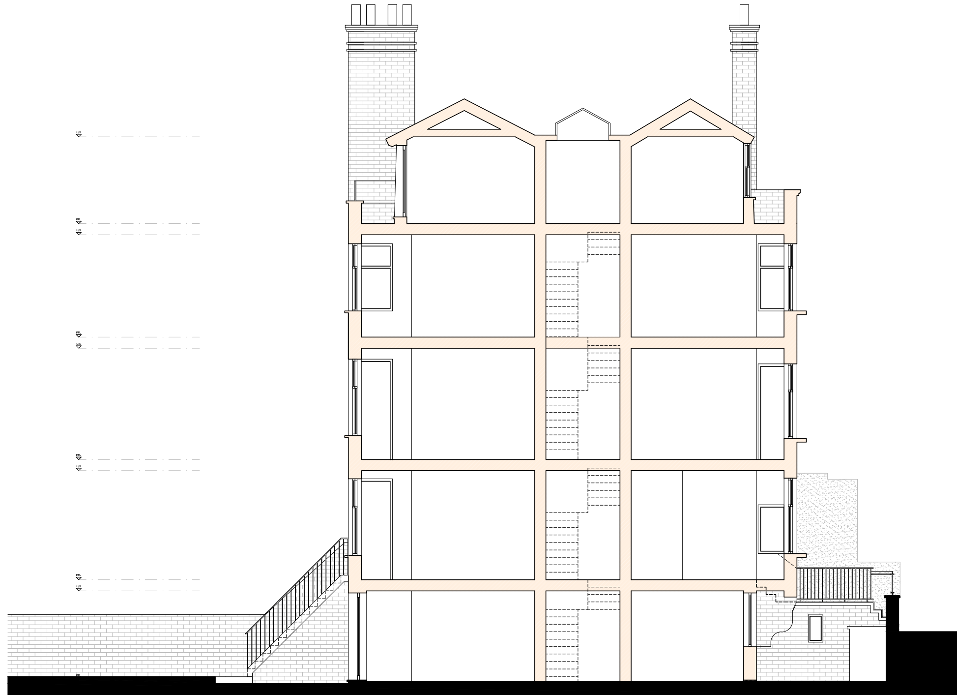
01 Existing Section AA 1:100 @A3
