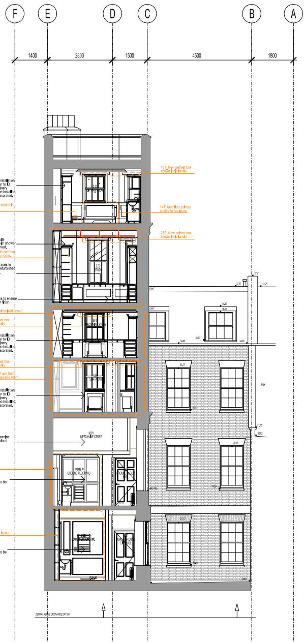
SECTION O - O
