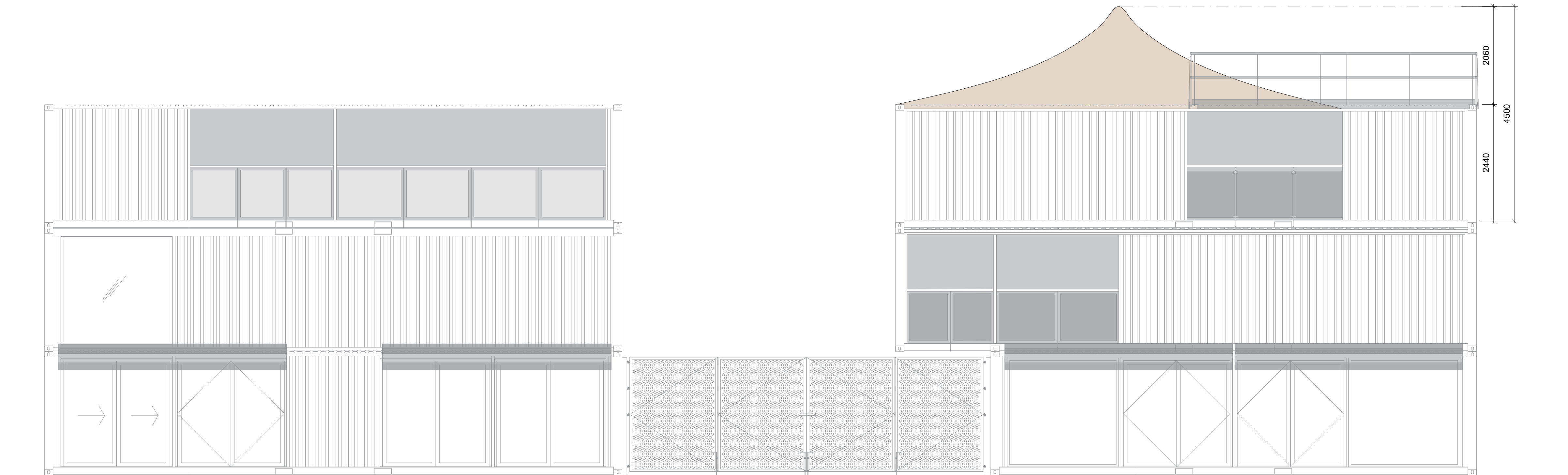
01 ELEVATION A-A SCALE 1:50 @ A1
