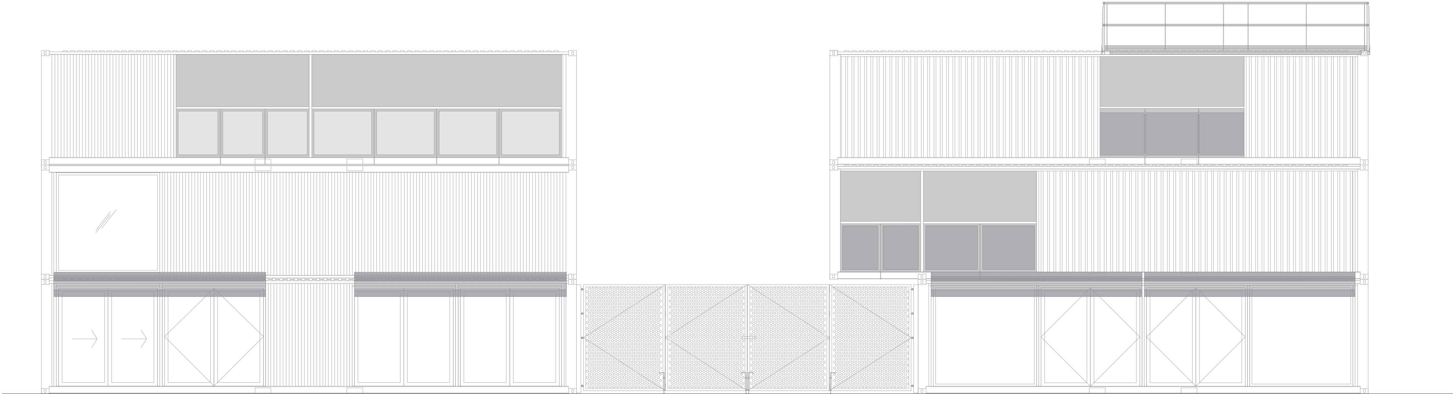
01 ELEVATION A-A SCALE 1:50 @ A1
