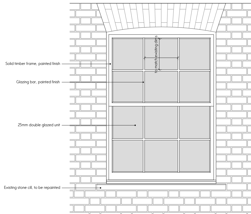
Elevation
