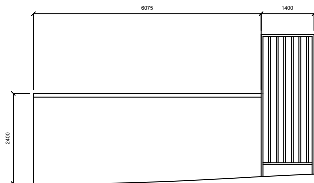
Elevation A
