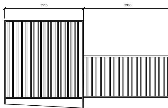
Elevation B
