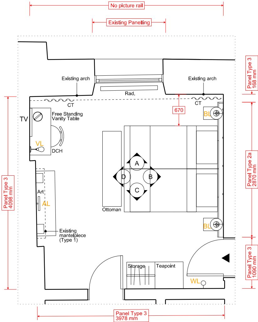
PLAN - 1:50 @ A3
