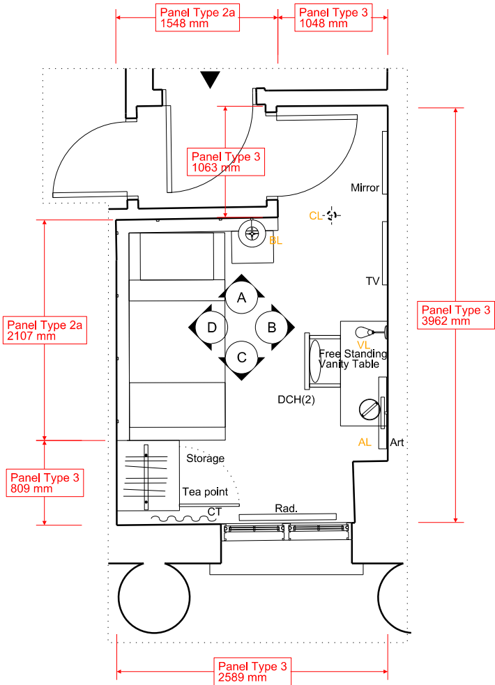
PLAN - 1:50 @ A3
