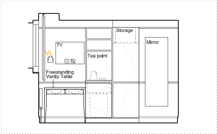
B - ELEVATION - 1:50 @ A3
