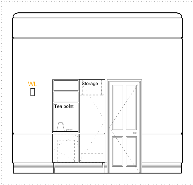
C - ELEVATION - 1:50 @ A3
