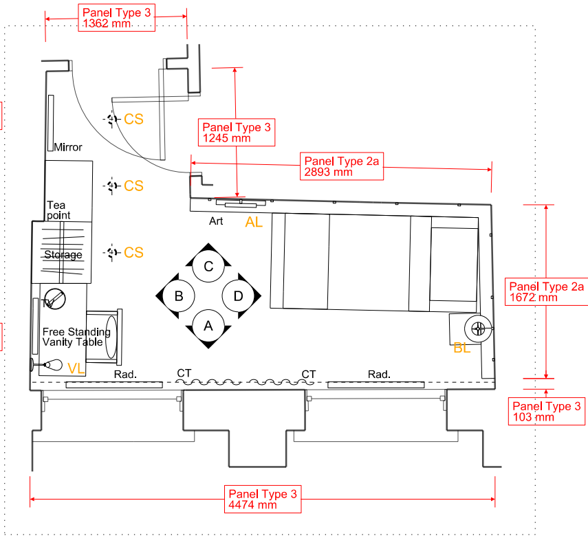
PLAN - 1:50 @ A3
