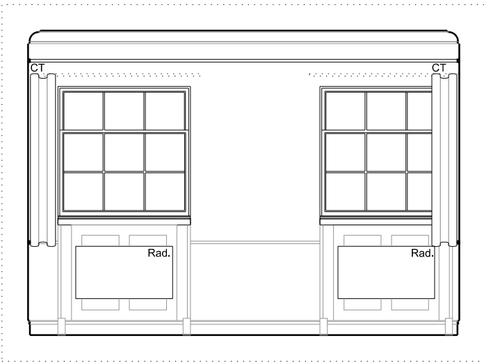
C - ELEVATION - 1:50 @ A3
