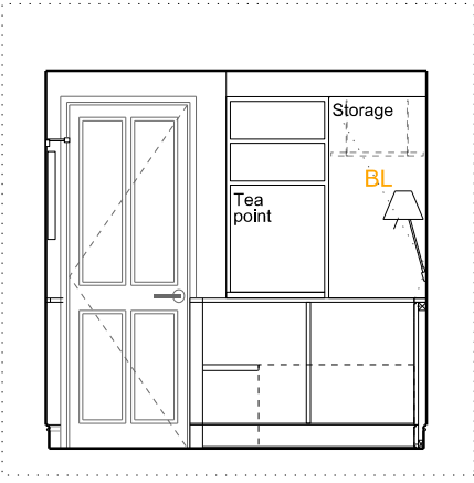
C - ELEVATION - 1:50 @ A3
