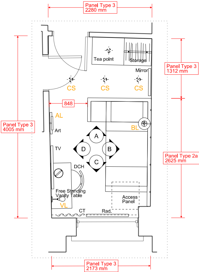
PLAN - 1:50 @ A3
