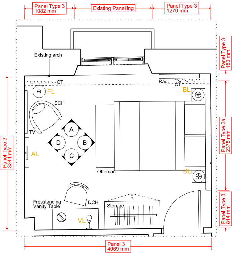
PLAN - 1:50 @ A3
