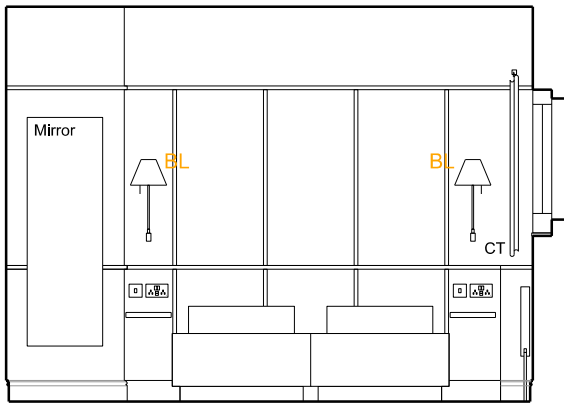
B - ELEVATION - 1:50 @ A3
