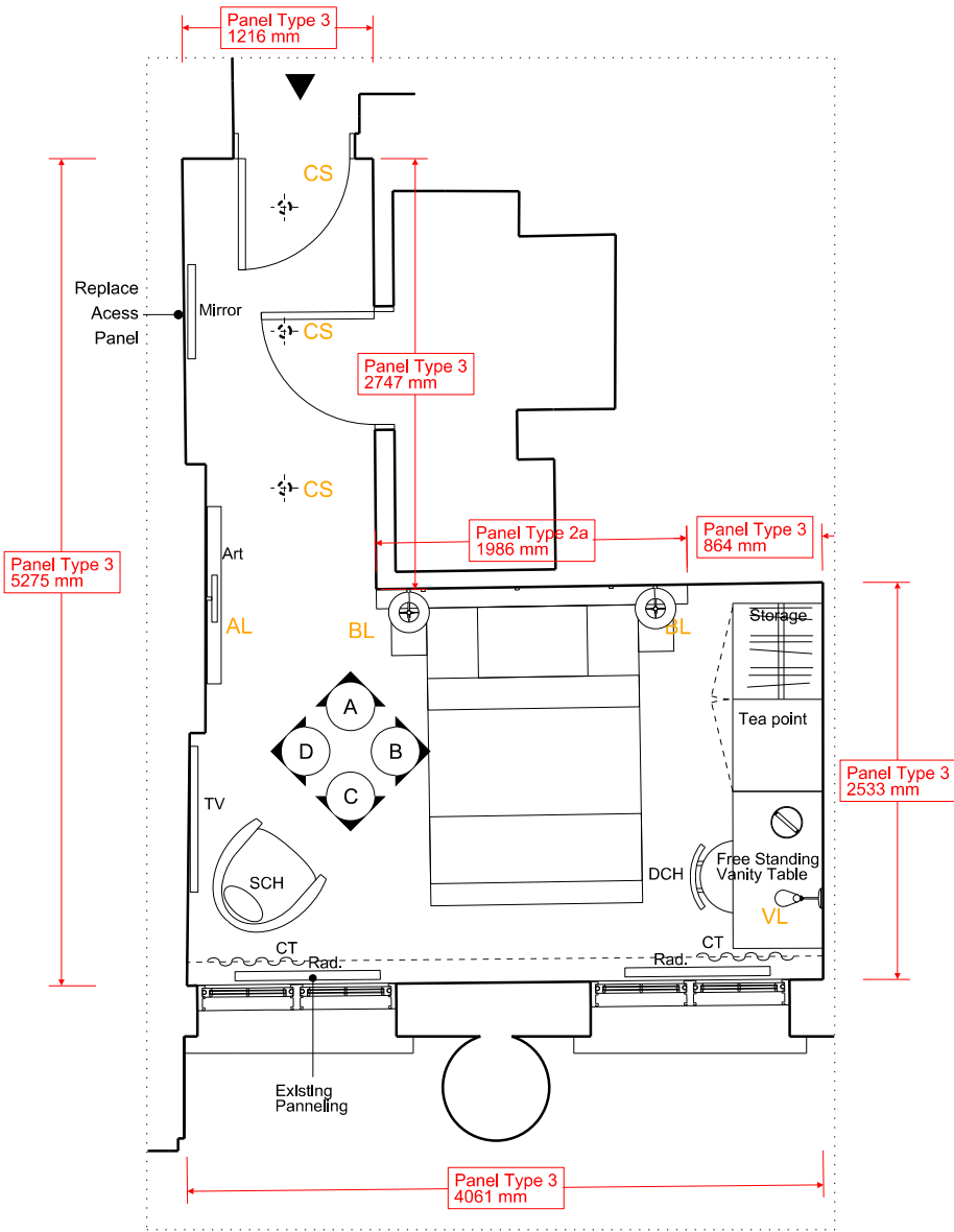
PLAN - 1:50 @ A3
