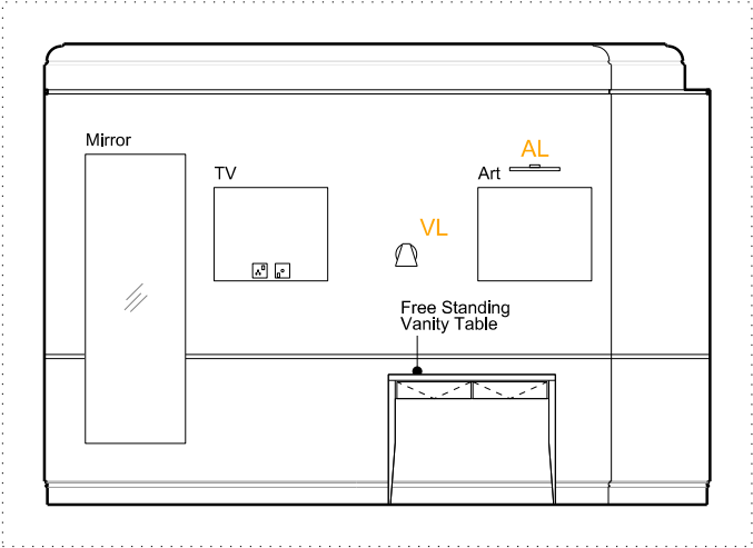
B - ELEVATION - 1:50 @ A3
