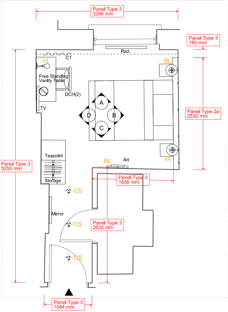
PLAN - 1:50 @ A3
