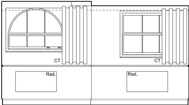
C - ELEVATION - 1:50 @ A3
