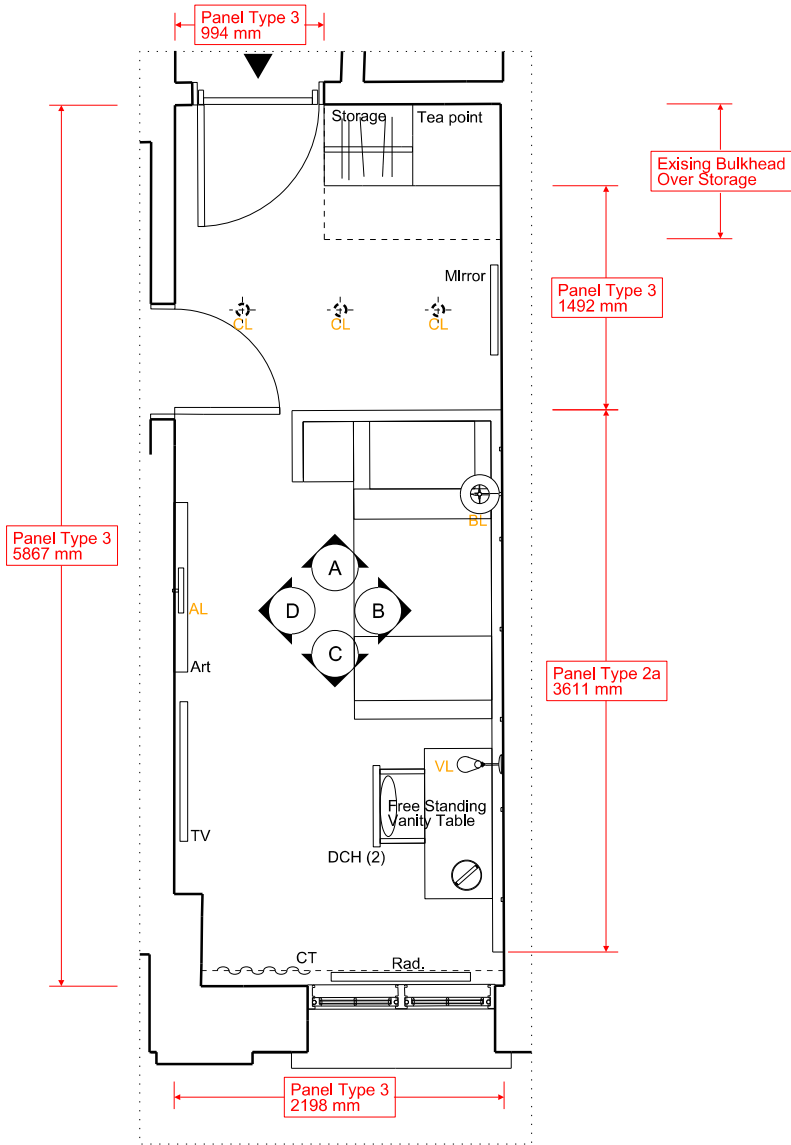
PLAN - 1:50 @ A3
