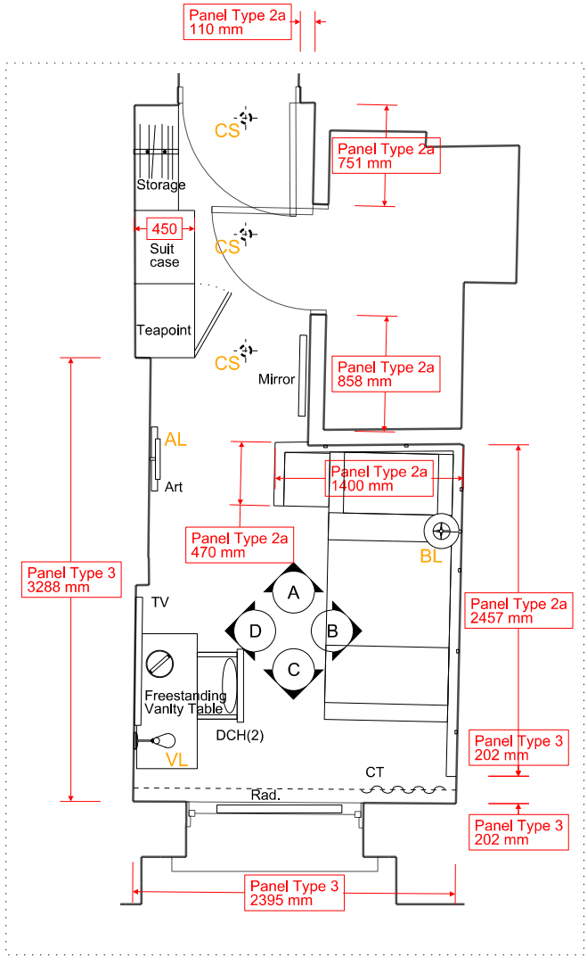
PLAN - 1:50 @ A3
