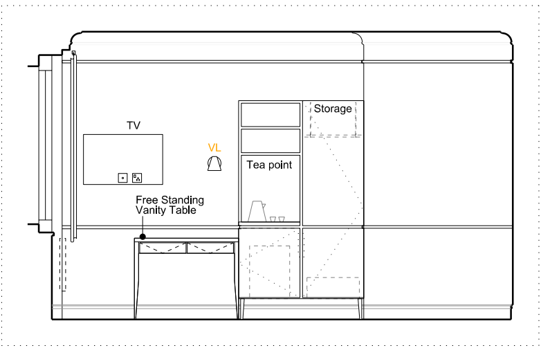
B - ELEVATION - 1:50 @ A3
