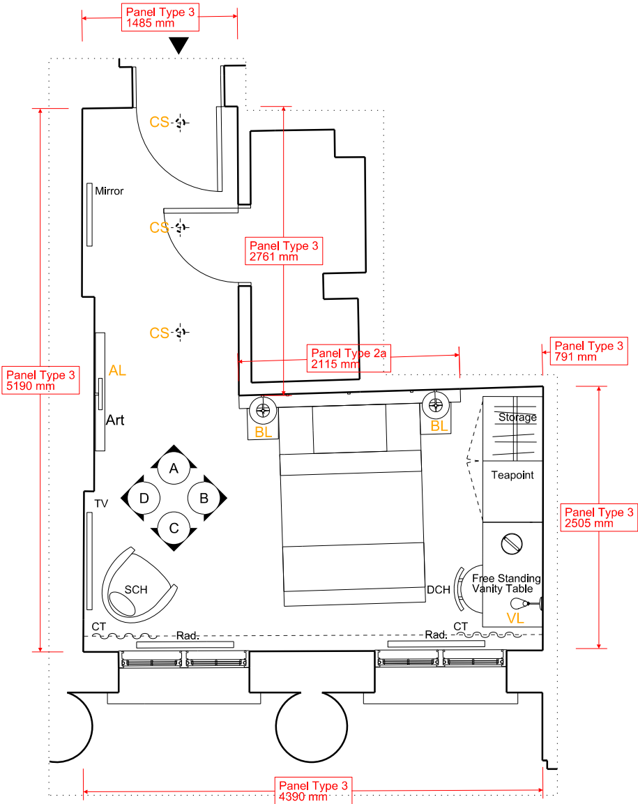
PLAN - 1:50 @ A3
