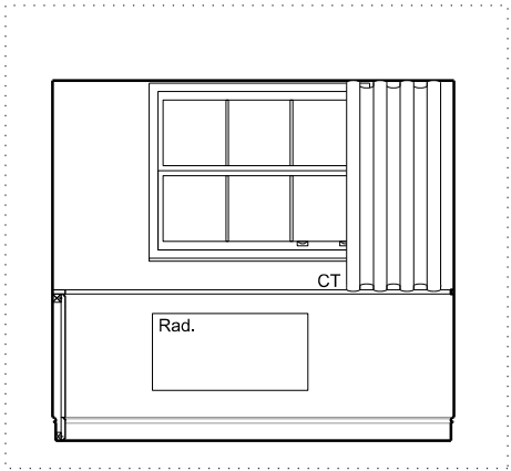
C - ELEVATION - 1:50 @ A3
