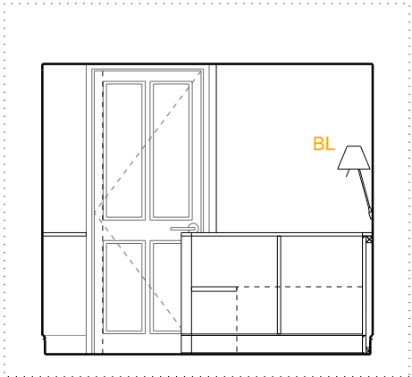
A - ELEVATION - 1:50 @ A3
