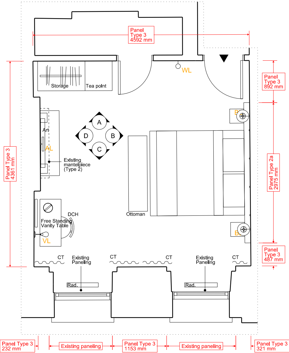
PLAN - 1:50 @ A3
