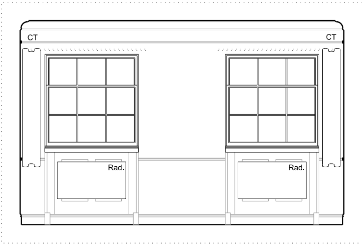
C - ELEVATION - 1:50 @ A3
