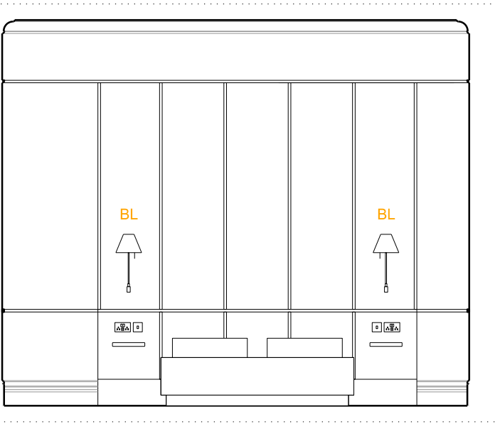
B - ELEVATION - 1:50 @ A3
