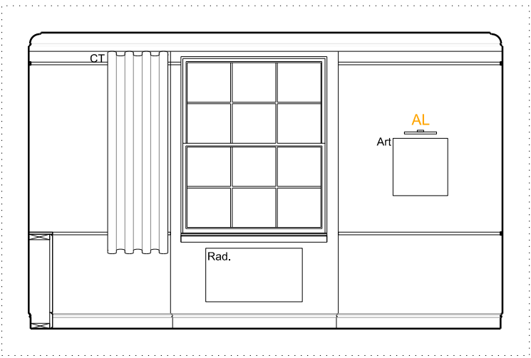
A - ELEVATION - 1:50 @ A3
