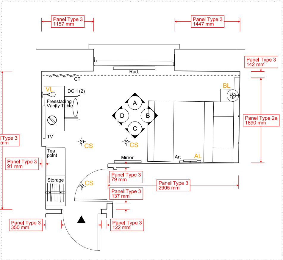
PLAN - 1:50 @ A3
