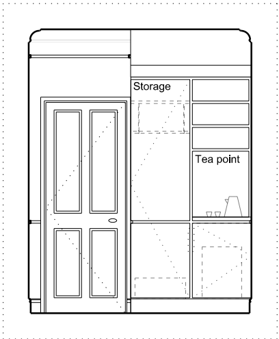
A - ELEVATION - 1:50 @ A3
