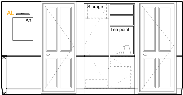
A - ELEVATION - 1:50 @ A3
