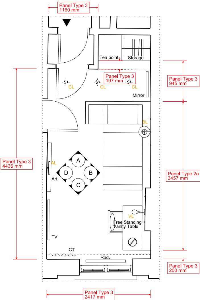
PLAN - 1:50 @ A3
