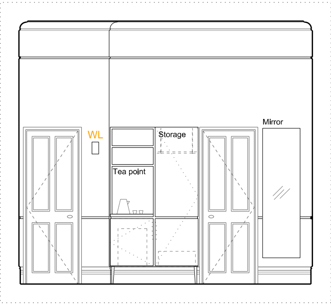
C - ELEVATION - 1:50 @ A3
