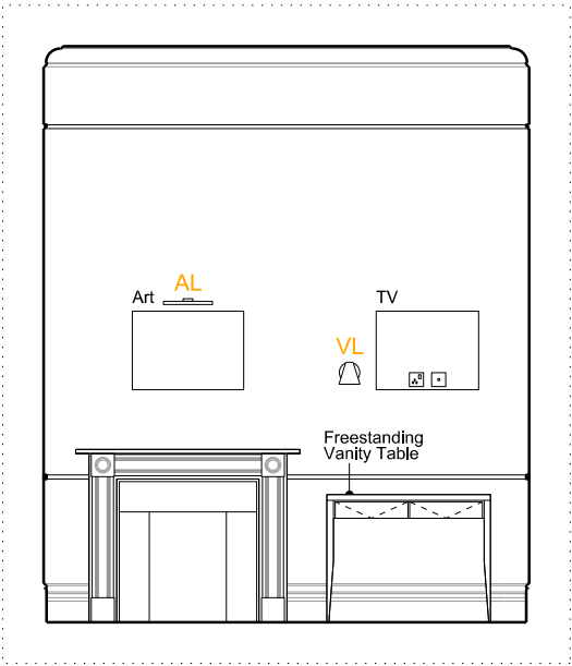
D - ELEVATION - 1:50 @ A3
