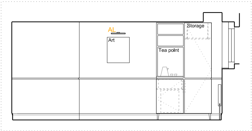
D - ELEVATION - 1:50 @ A3
