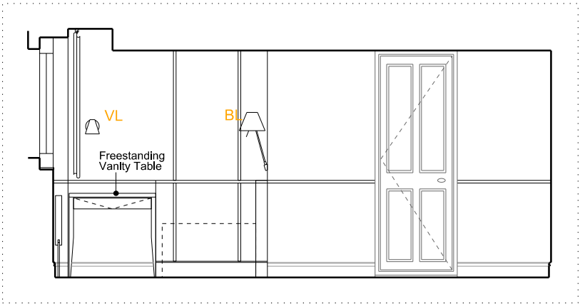
B - ELEVATION - 1:50 @ A3
