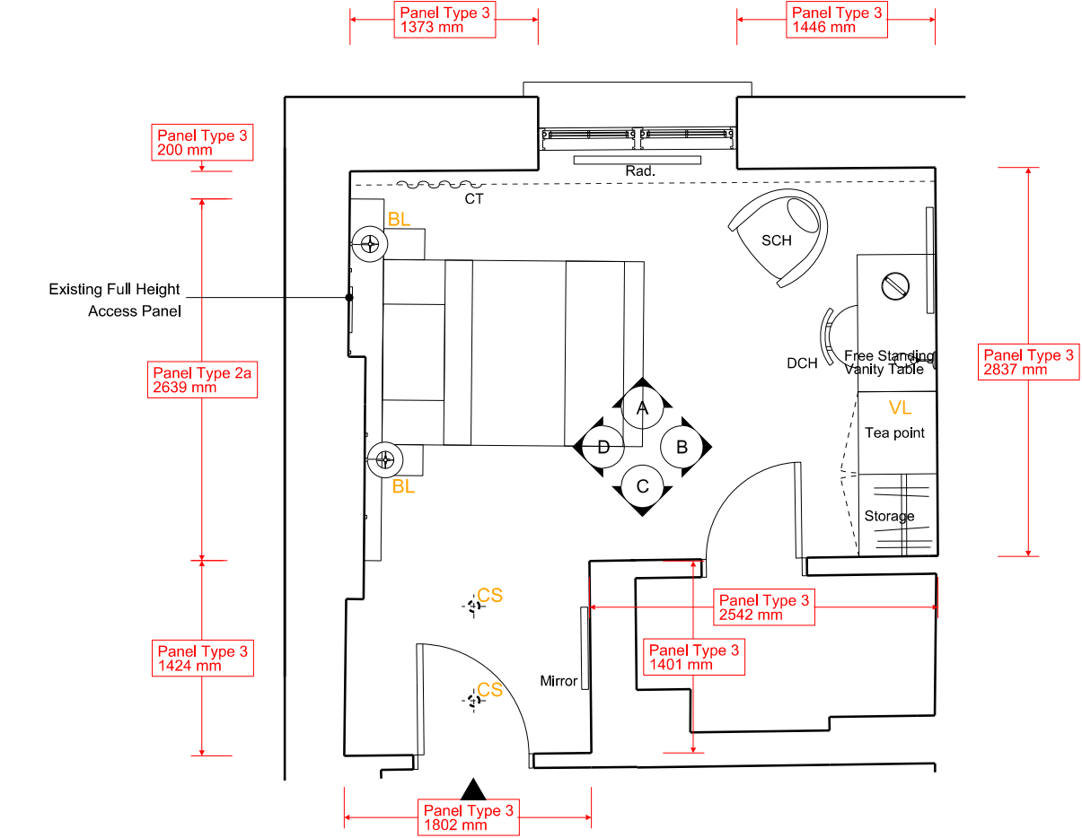
PLAN - 1:50 @ A3
