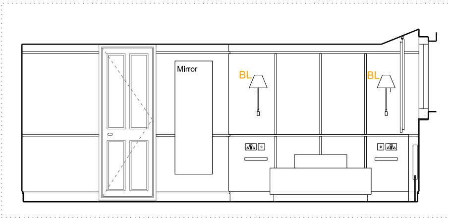
B - ELEVATION - 1:50 @ A3
