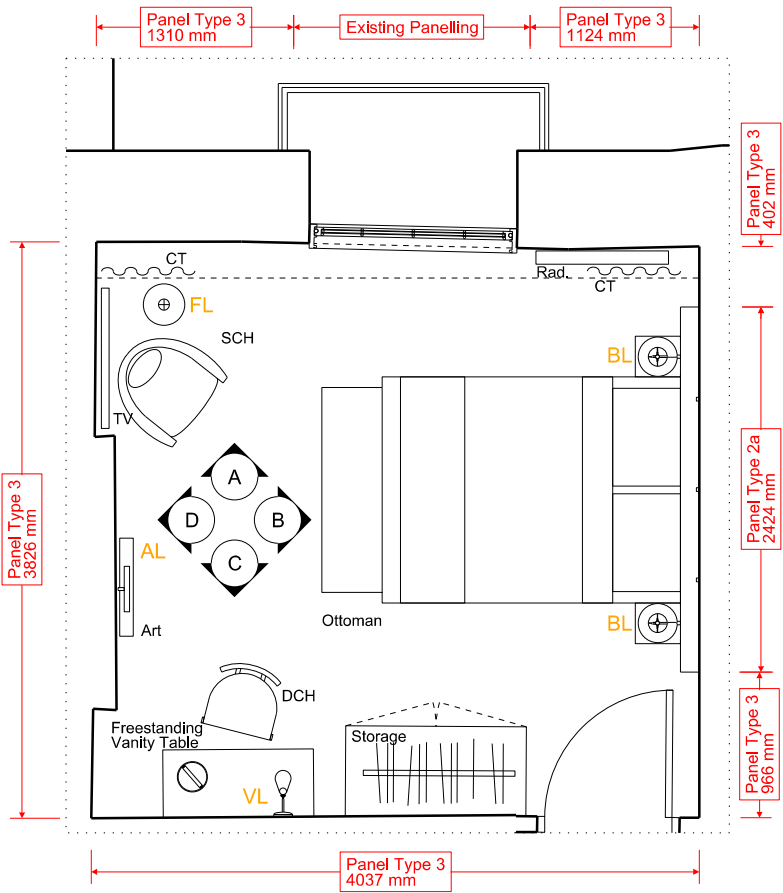
PLAN - 1:50 @ A3
