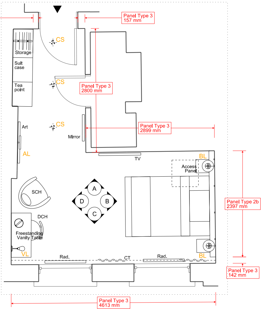
PLAN - 1:50 @ A3
