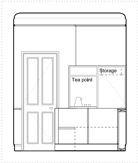
A - ELEVATION - 1:50 @ A3
