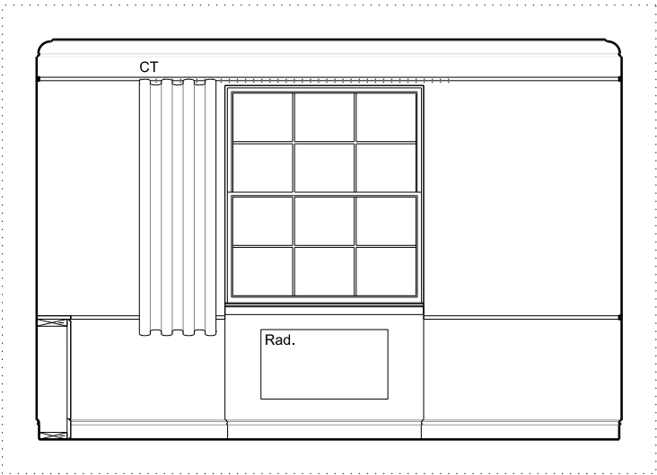
A - ELEVATION - 1:50 @ A3
