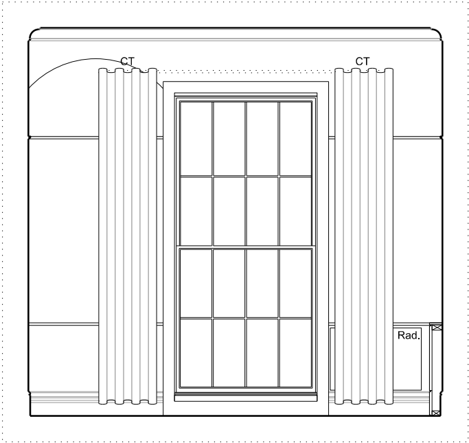
A - ELEVATION - 1:50 @ A3
