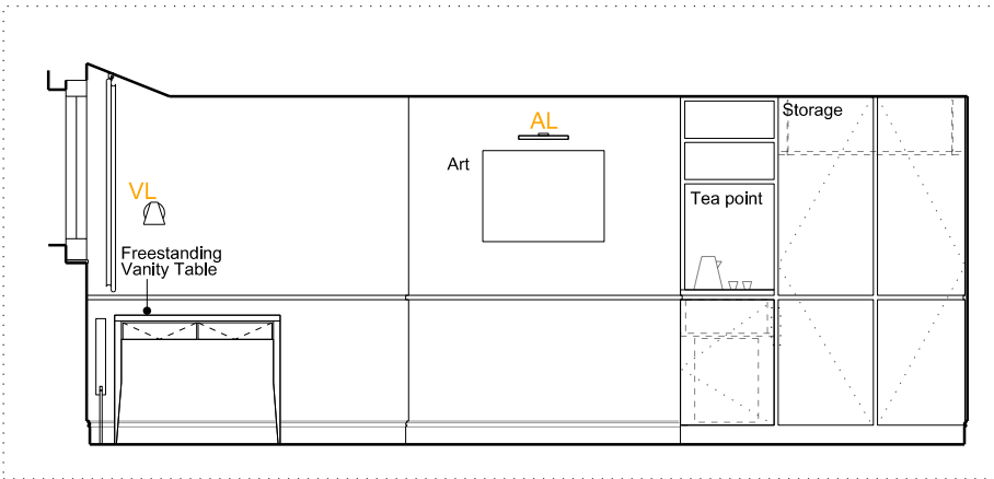
D - ELEVATION - 1:50 @ A3
