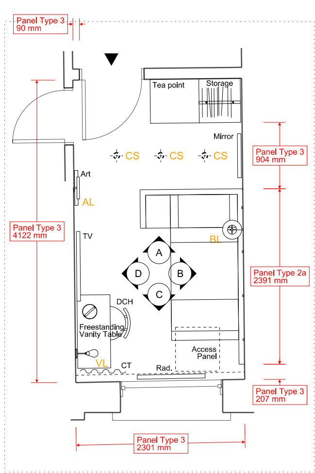
PLAN - 1:50 @ A3
