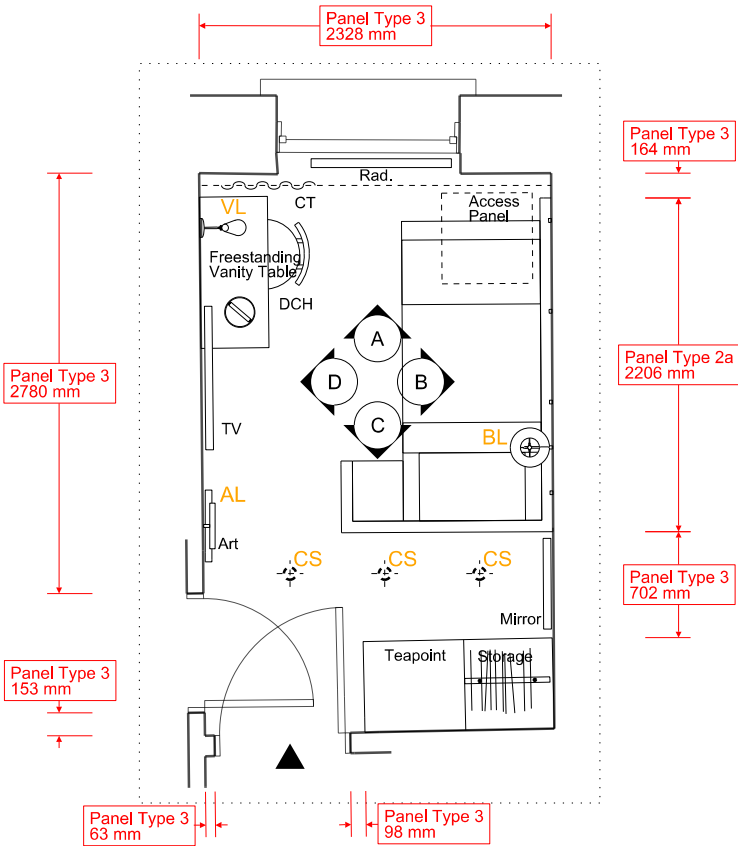
PLAN - 1:50 @ A3
