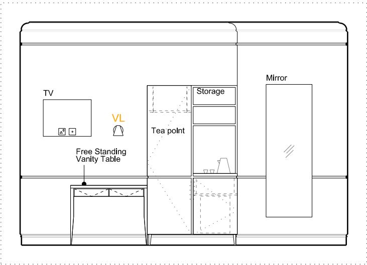
B - ELEVATION - 1:50 @ A3
