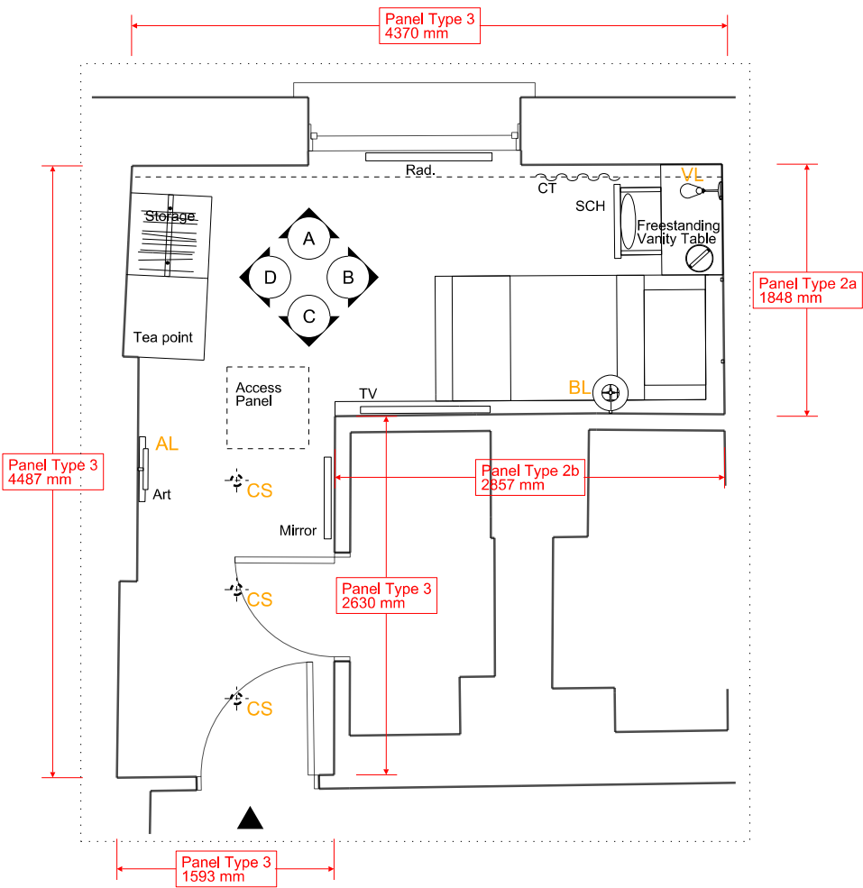
PLAN - 1:50 @ A3
