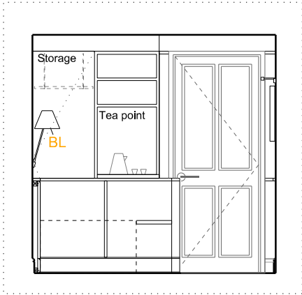
C - ELEVATION - 1:50 @ A3
