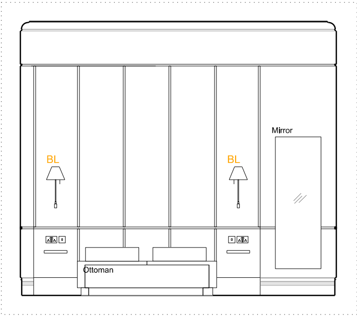
B - ELEVATION - 1:50 @ A3
