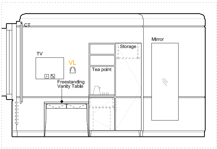
B - ELEVATION - 1:50 @ A3
