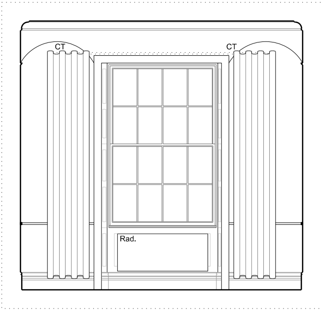
A - ELEVATION - 1:50 @ A3
