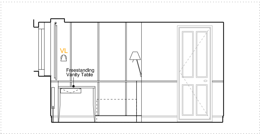
B - ELEVATION - 1:50 @ A3
