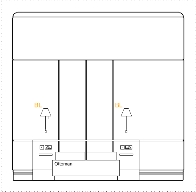
B - ELEVATION - 1:50 @ A3
