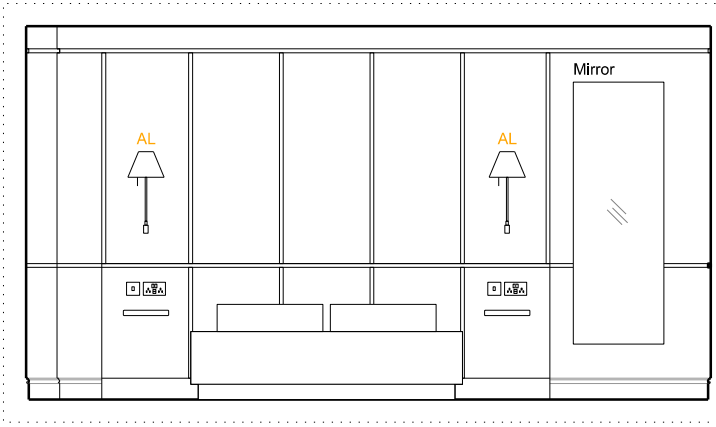
B - ELEVATION - 1:50 @ A3
