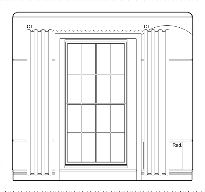
A - ELEVATION - 1:50 @ A3
