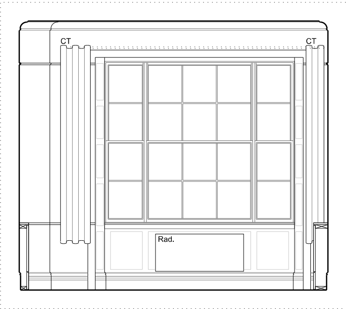
C - ELEVATION - 1:50 @ A3
