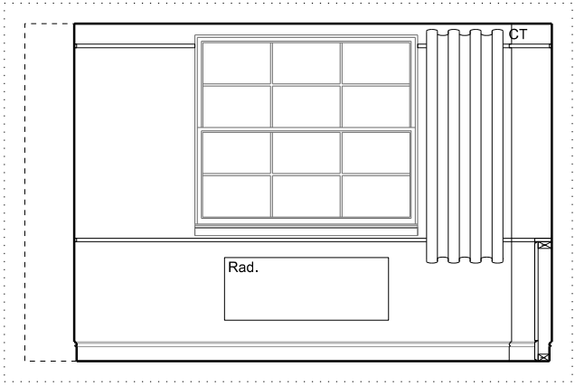
A - ELEVATION - 1:50 @ A3
