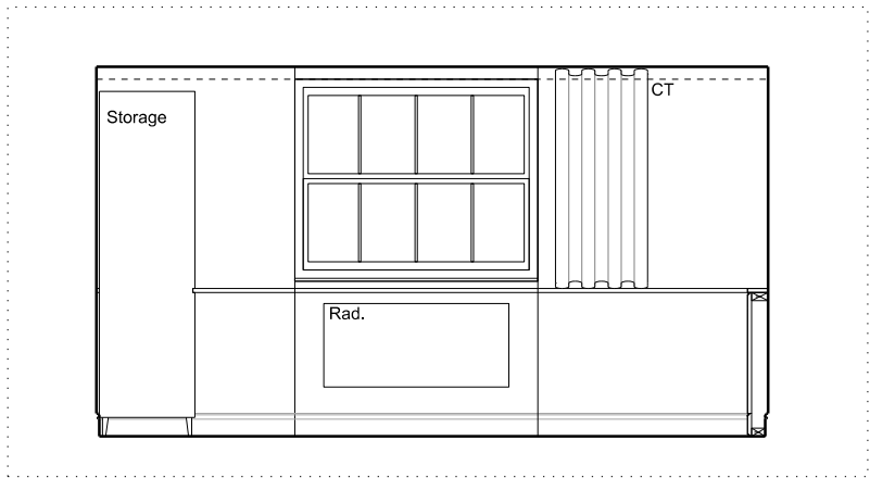
A - ELEVATION - 1:50 @ A3
