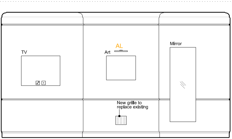
D - ELEVATION - 1:50 @ A3
