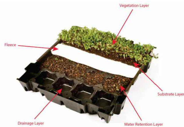
Sedum Pod Build up
