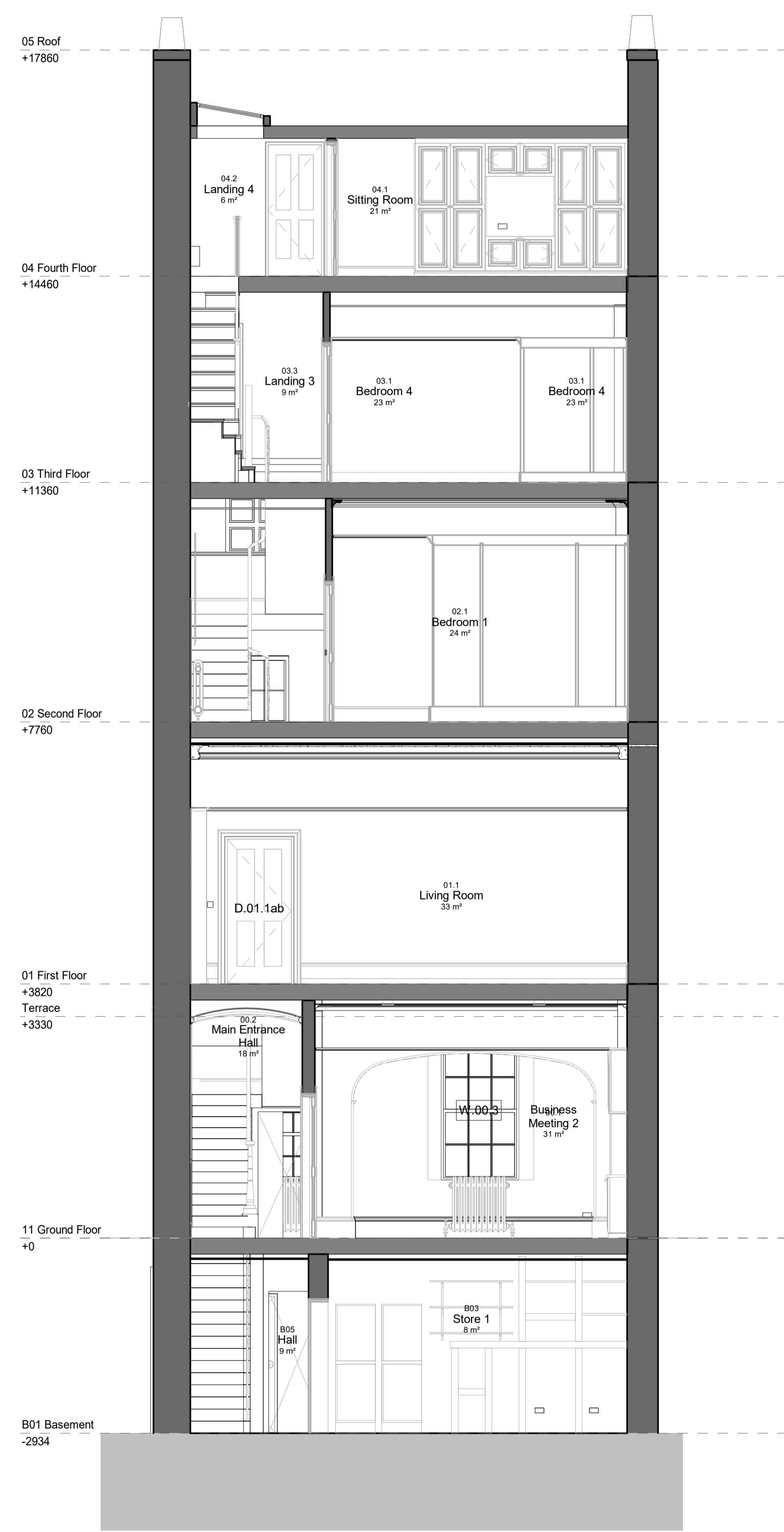
Section C Scale 1 : 50
