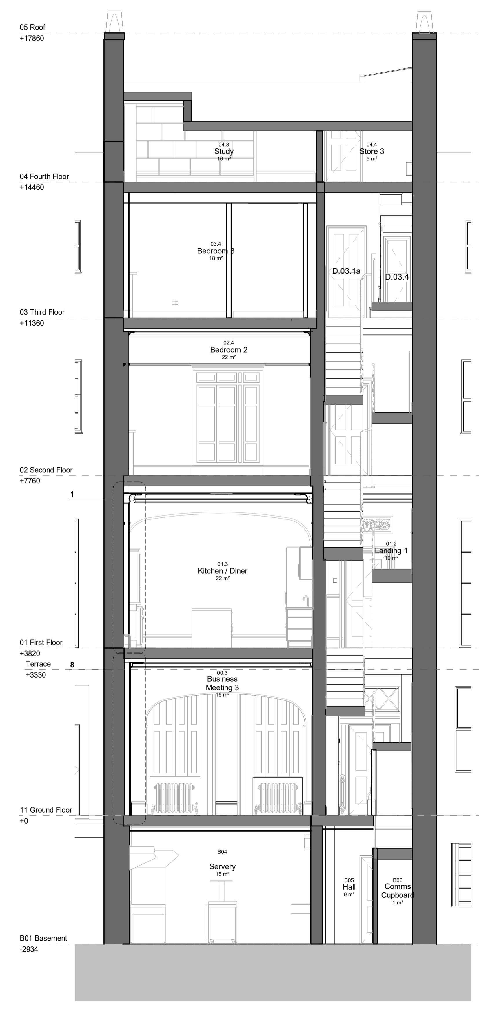
Section D Scale 1 : 50
