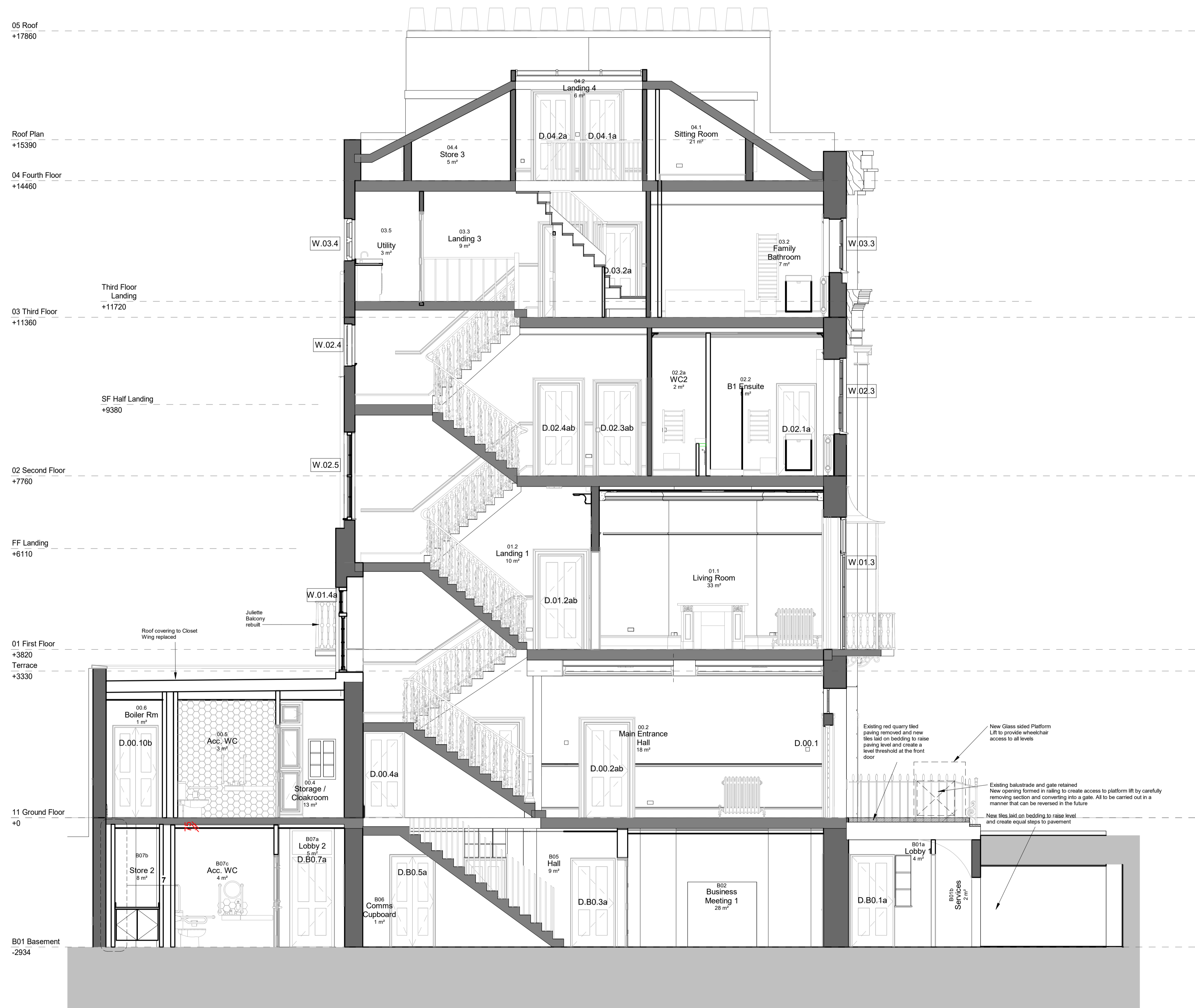
Section A Scale 1 : 50
