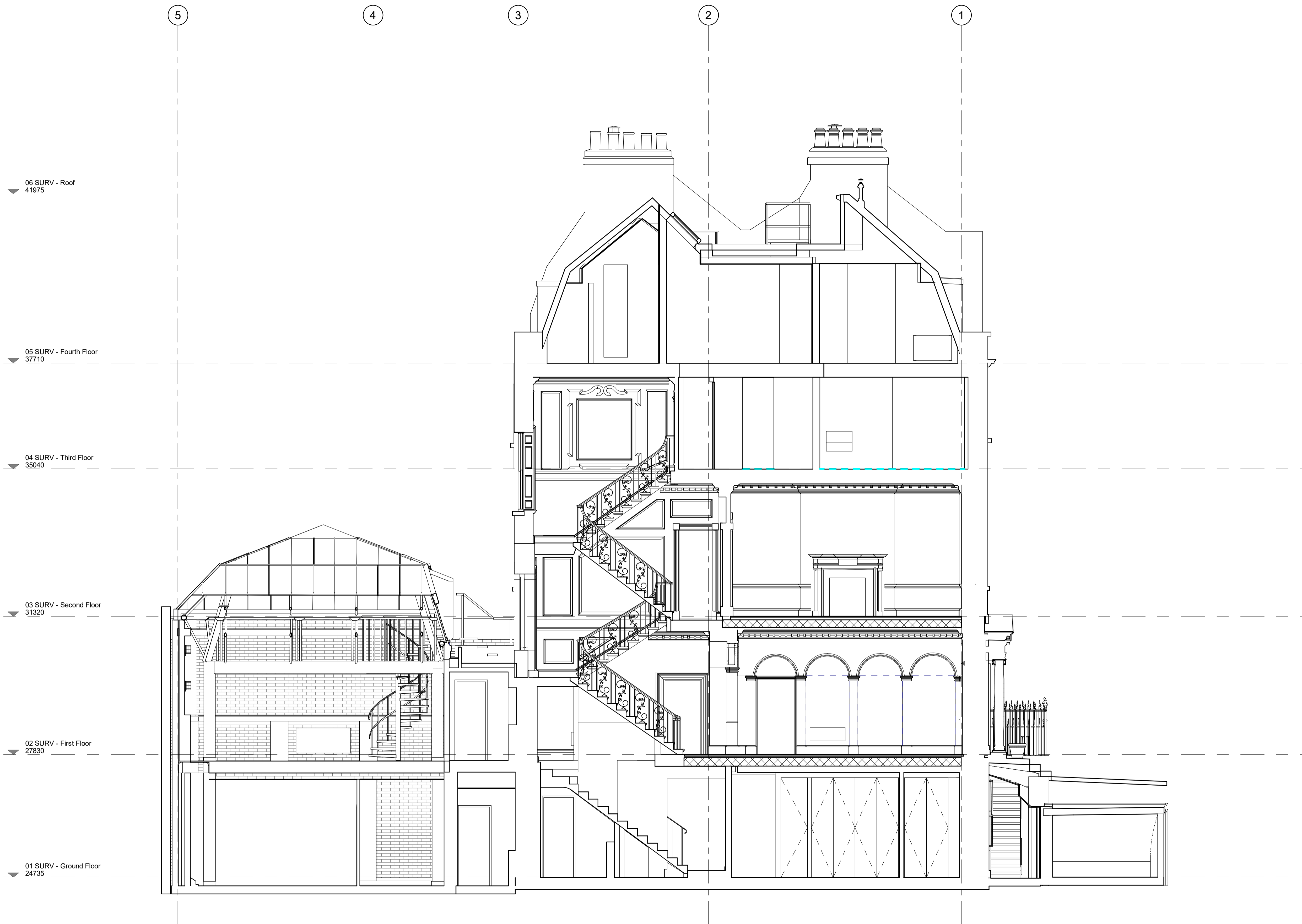
Existing Section S1 1 : 50
