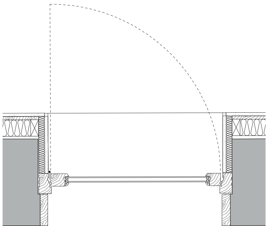
DOOR TYPE 01: HARDWOOD FRAME DOOR
