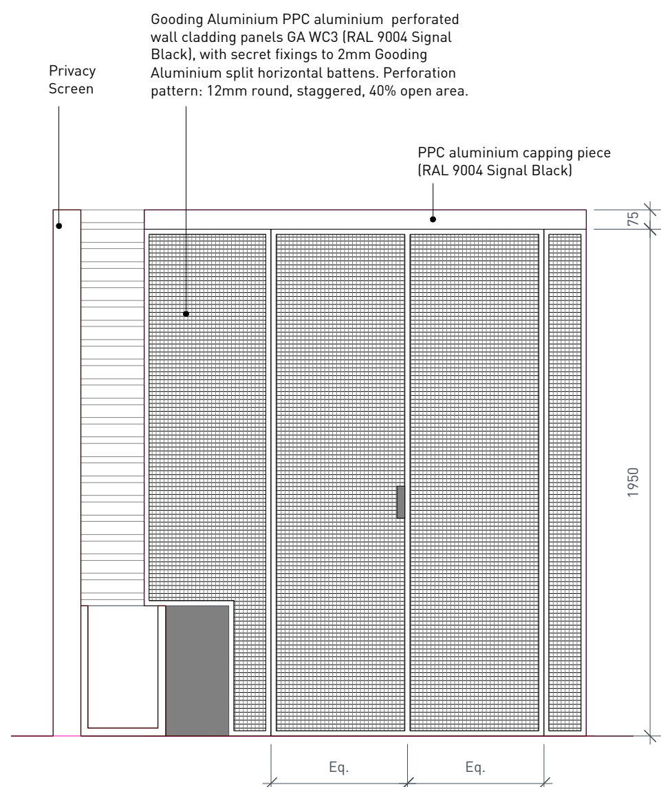
ELEVATION 02 1:20 @ A1
