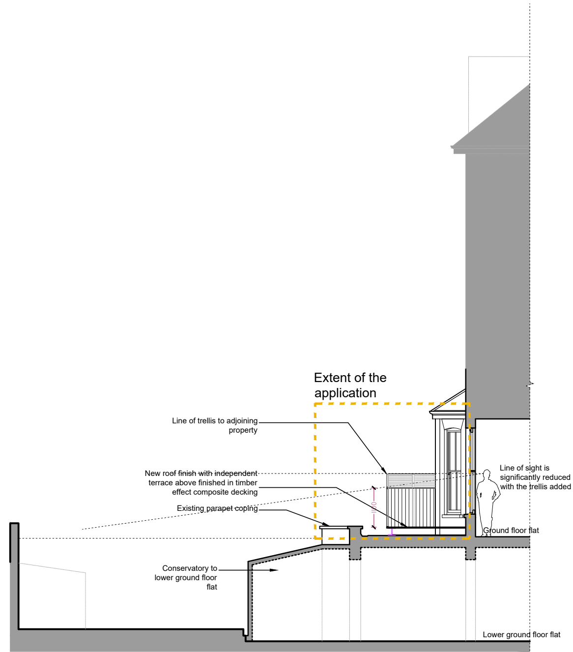
Section A-A
