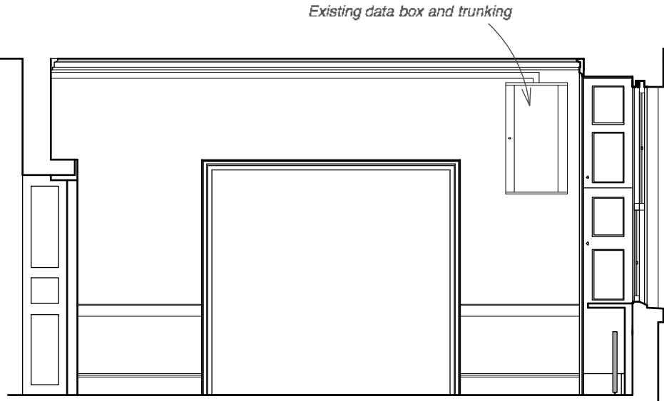
ELEVATION 4
