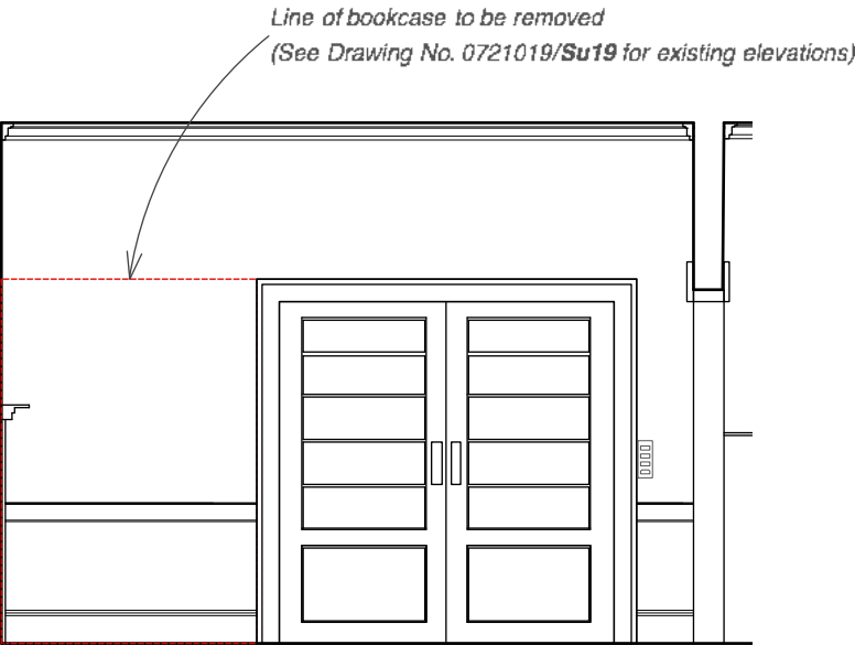
ELEVATION 3
