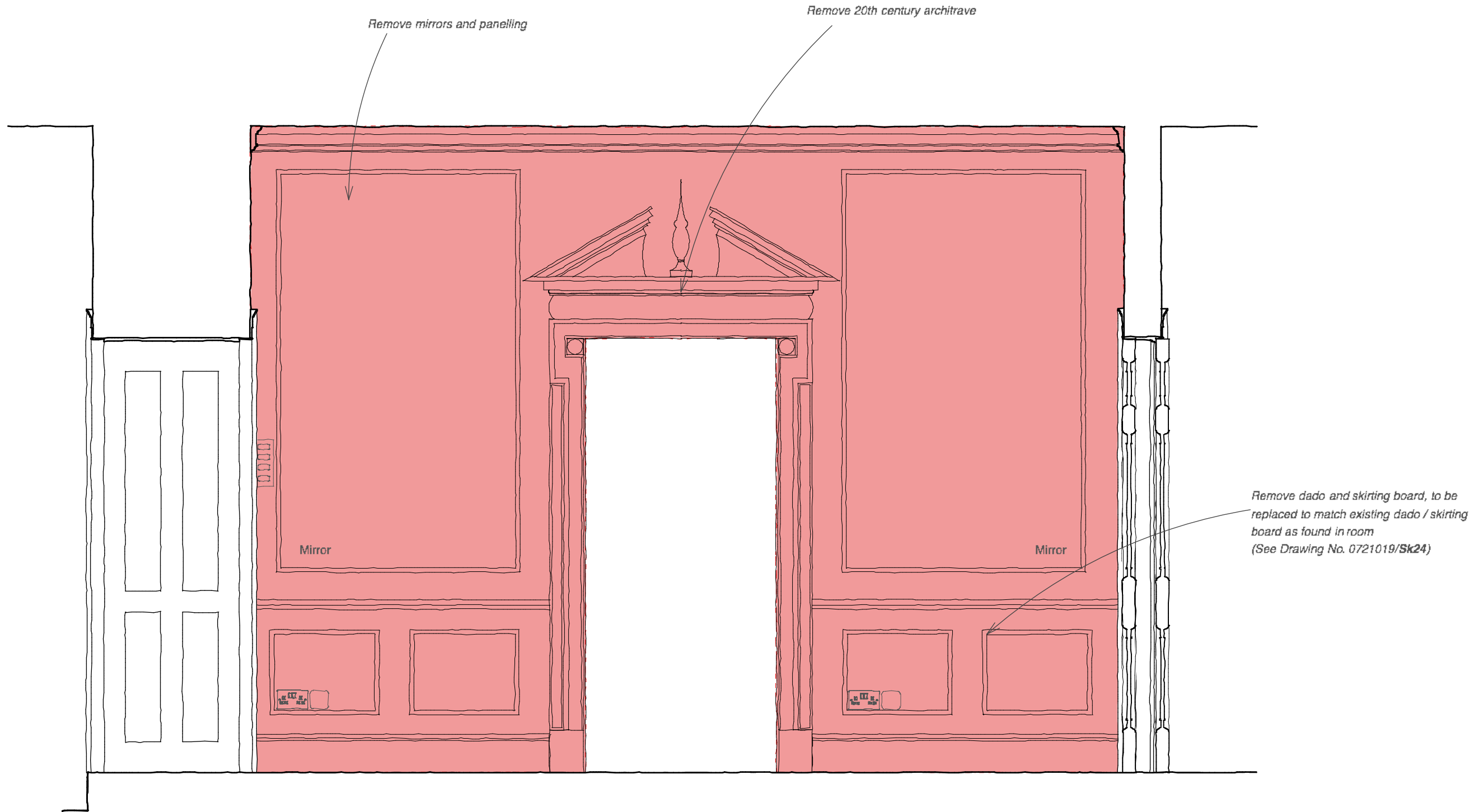
ELEVATION 1
