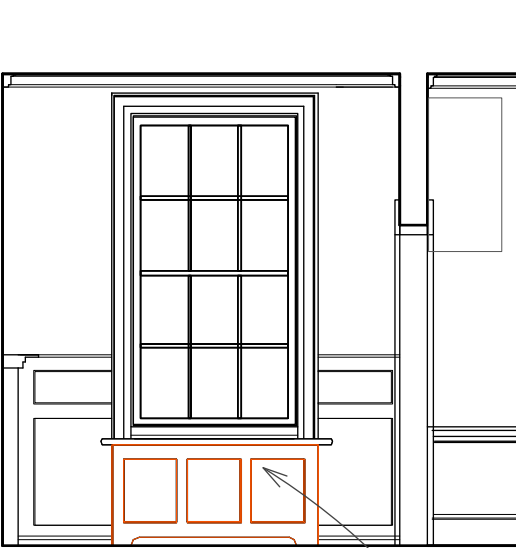
ELEVATION 1
