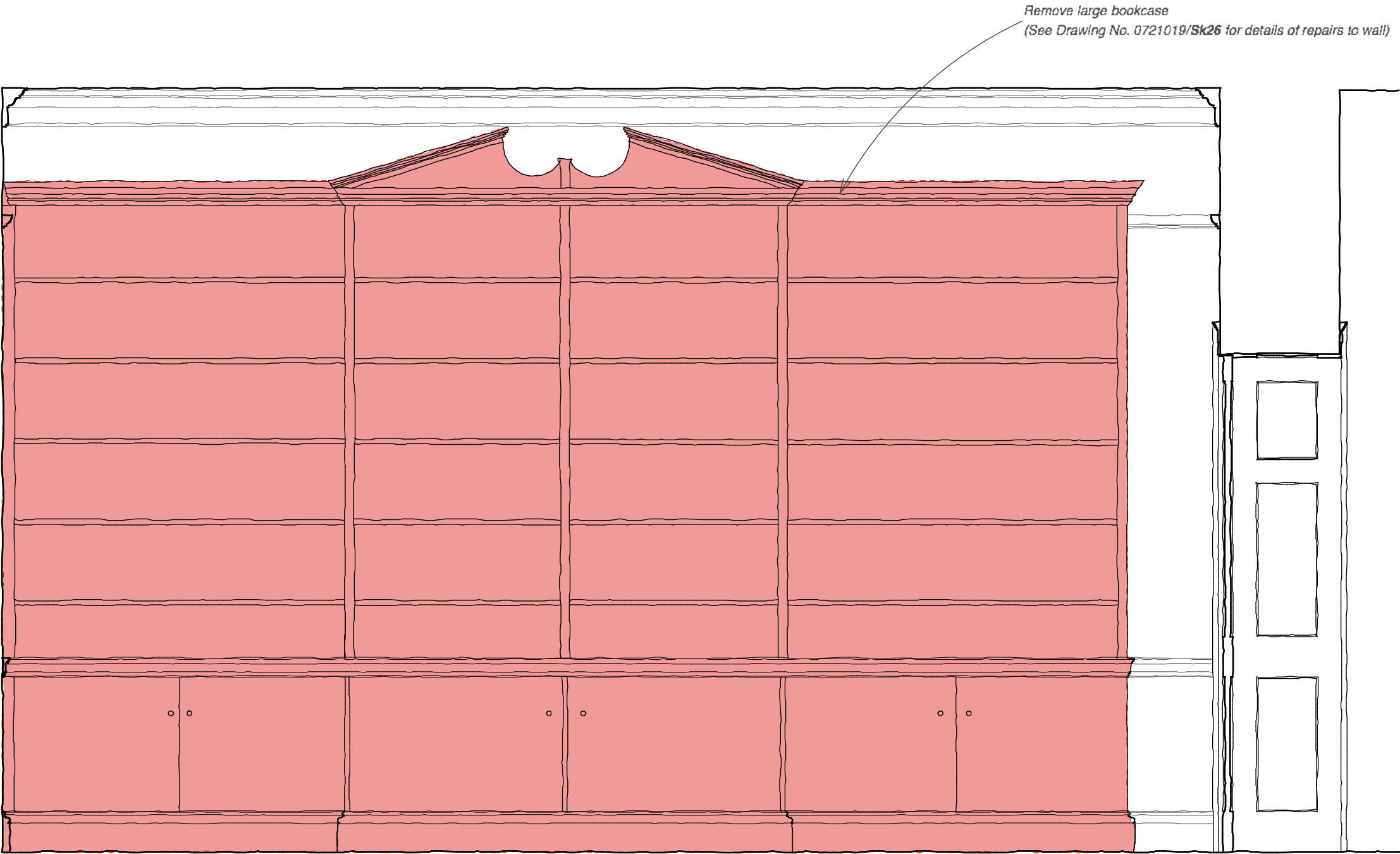
ELEVATION 3
