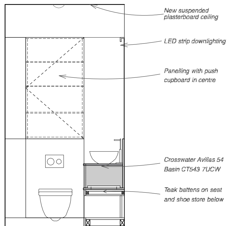
ELEVATION 1
