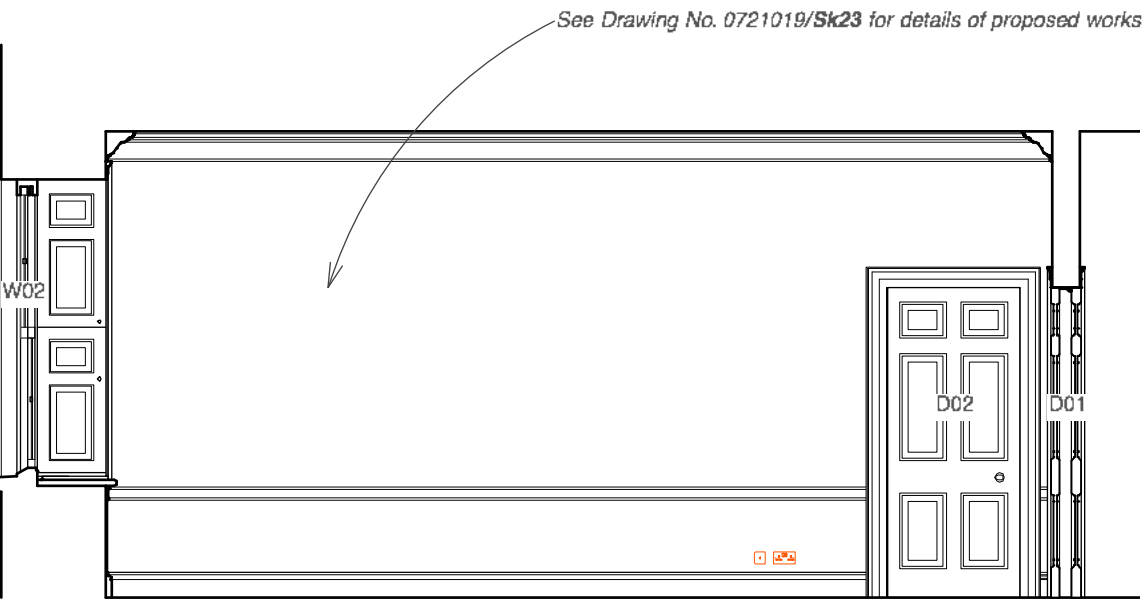
ELEVATION 3
