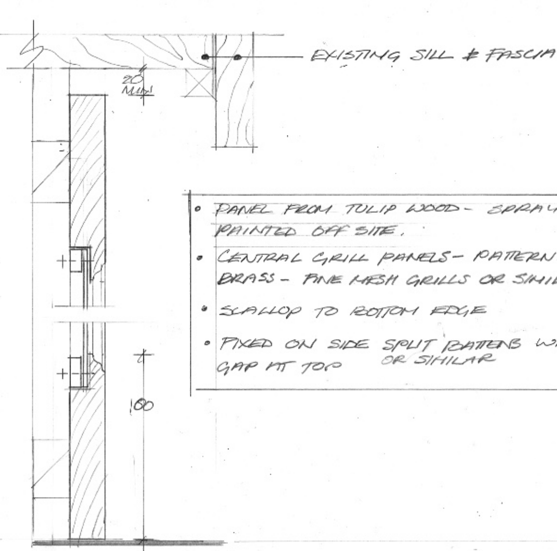
SECTION A 1:20 @ A4
