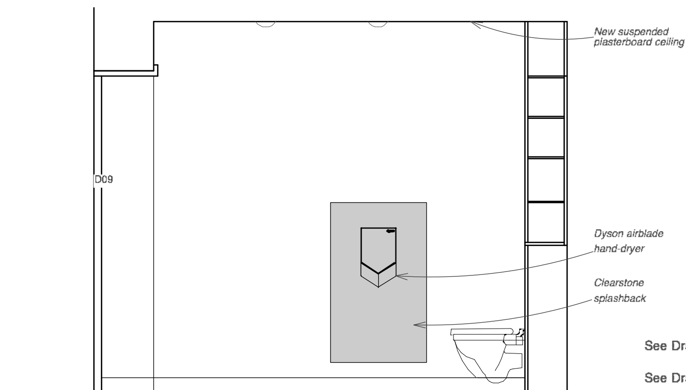
ELEVATION 2
