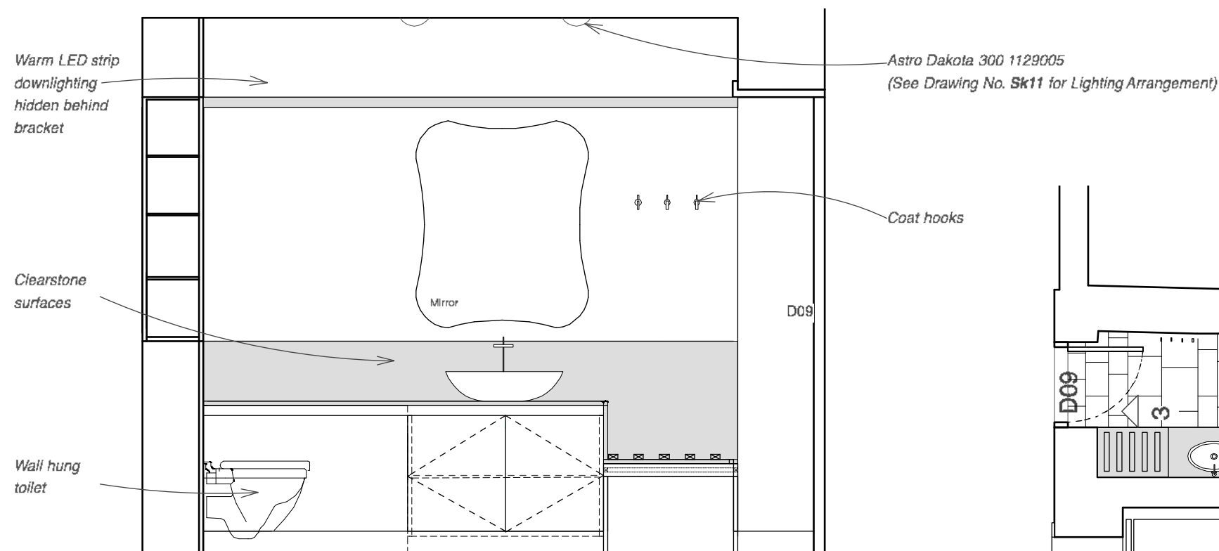
ELEVATION 2
