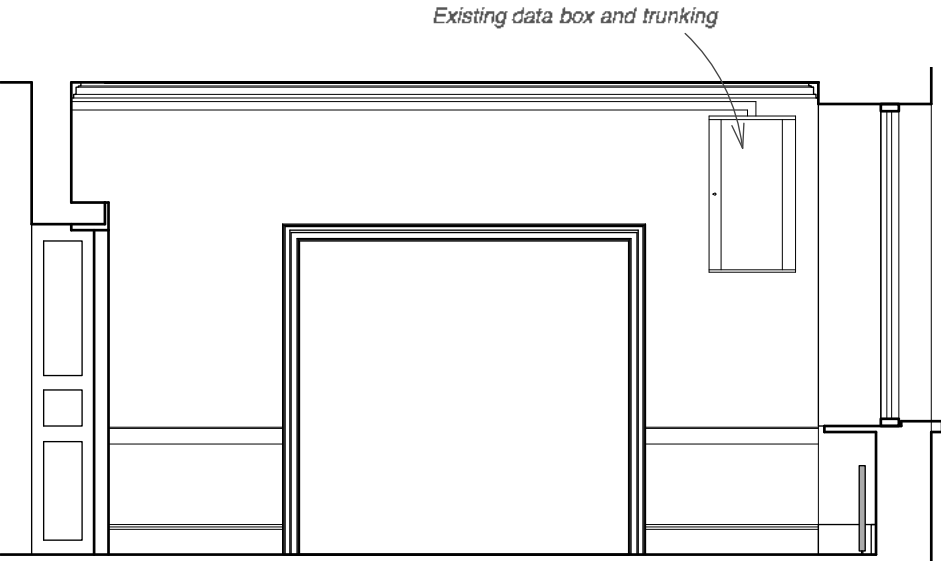
ELEVATION 4
