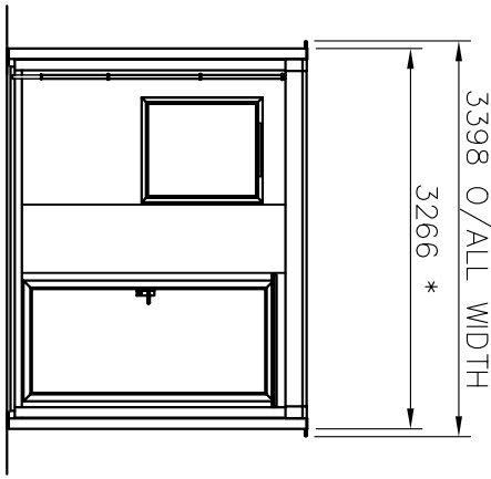
END ELEVATION
