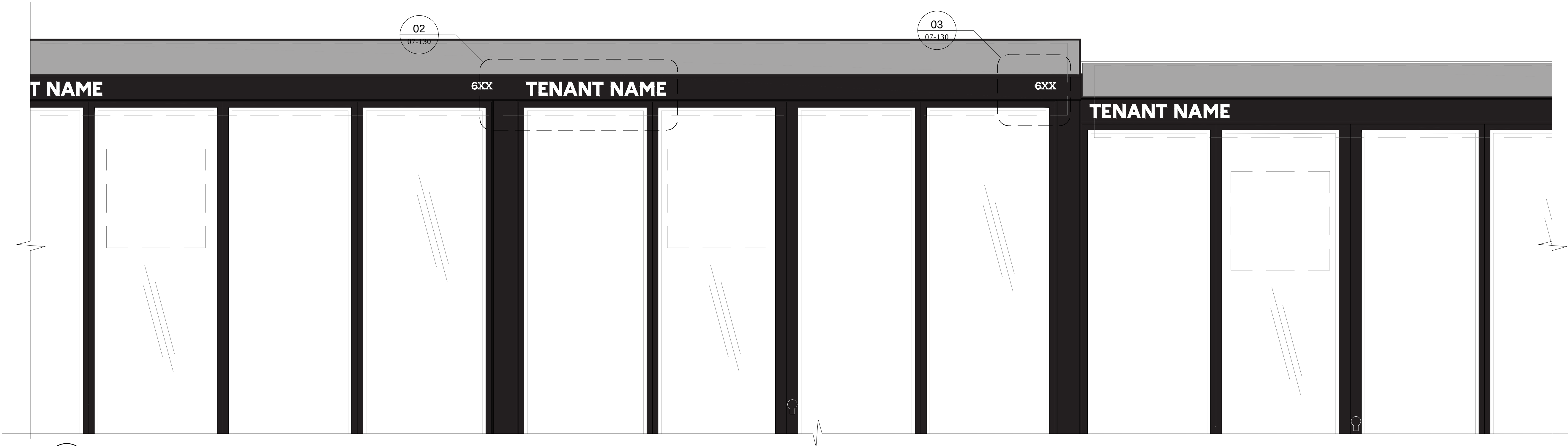
01 SIGNAGE-DETAIL 1 07-130 1:10
