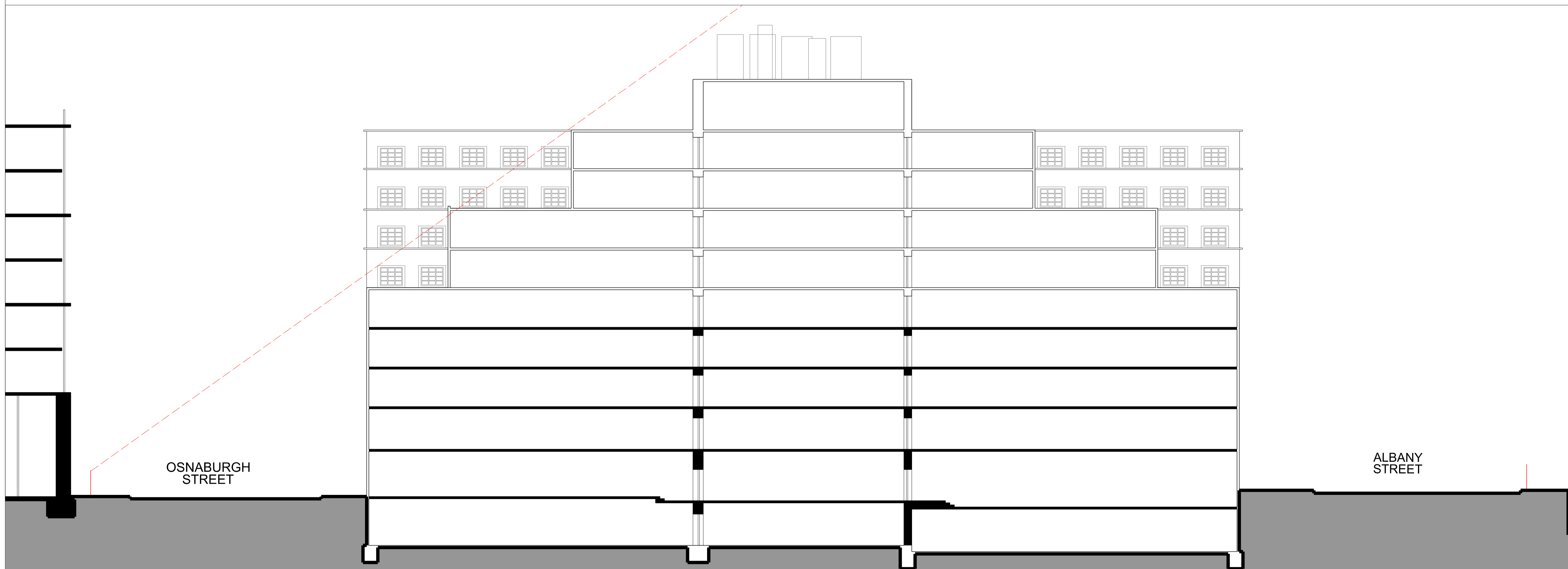
SECTION A-A'
