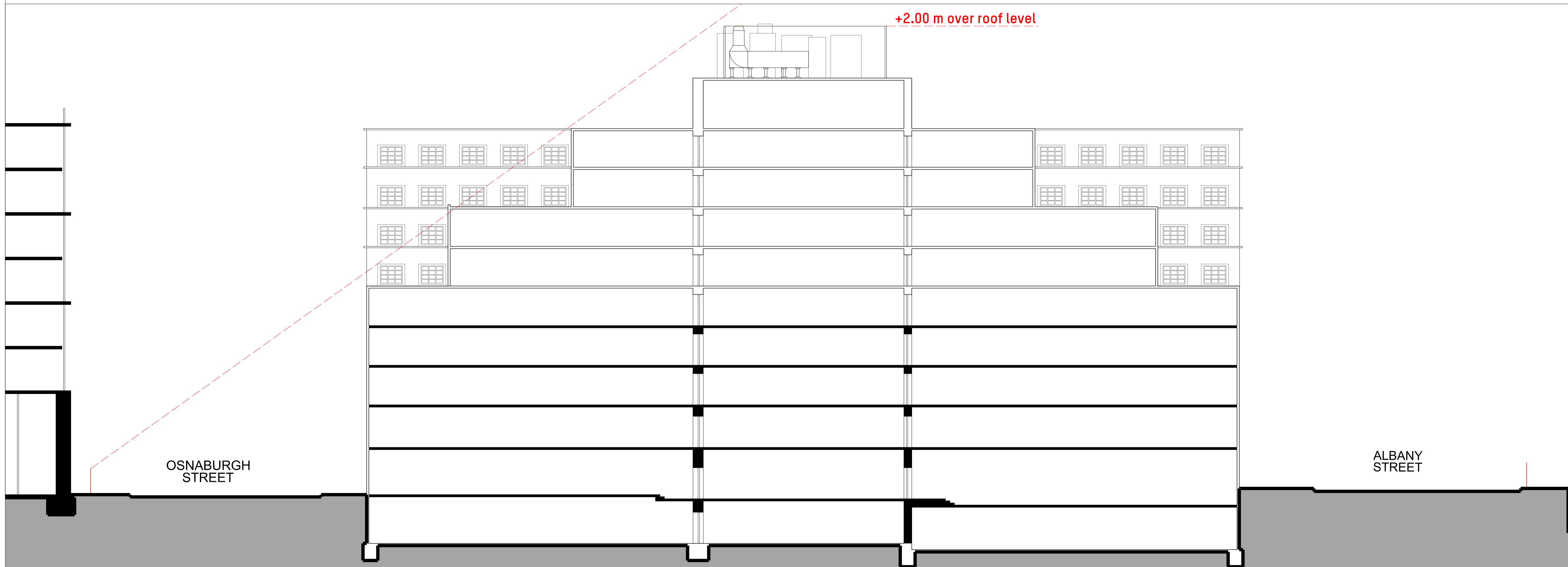
SECTION A-A'
