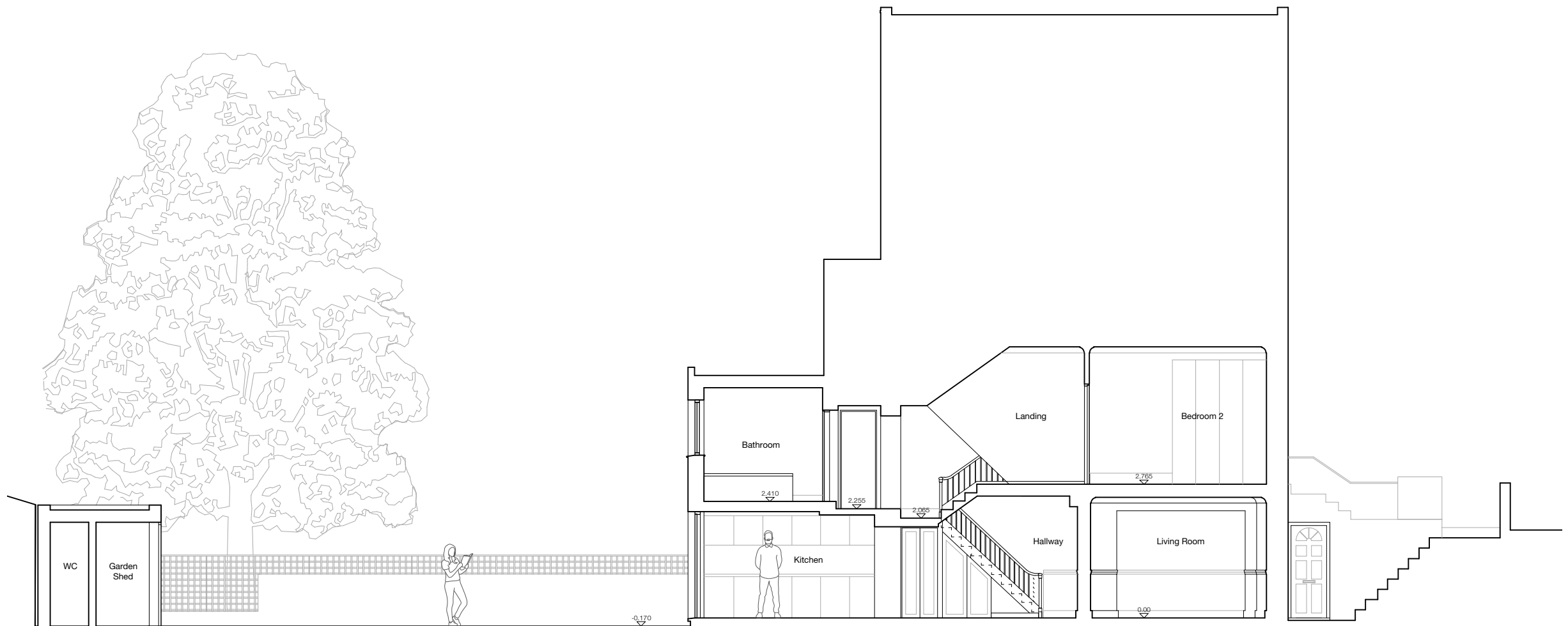
01 SECTION BB
