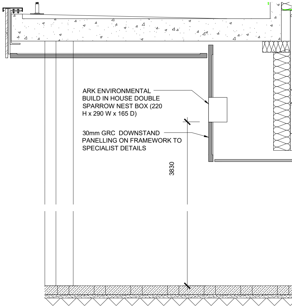
SECTION A-A 1:20
