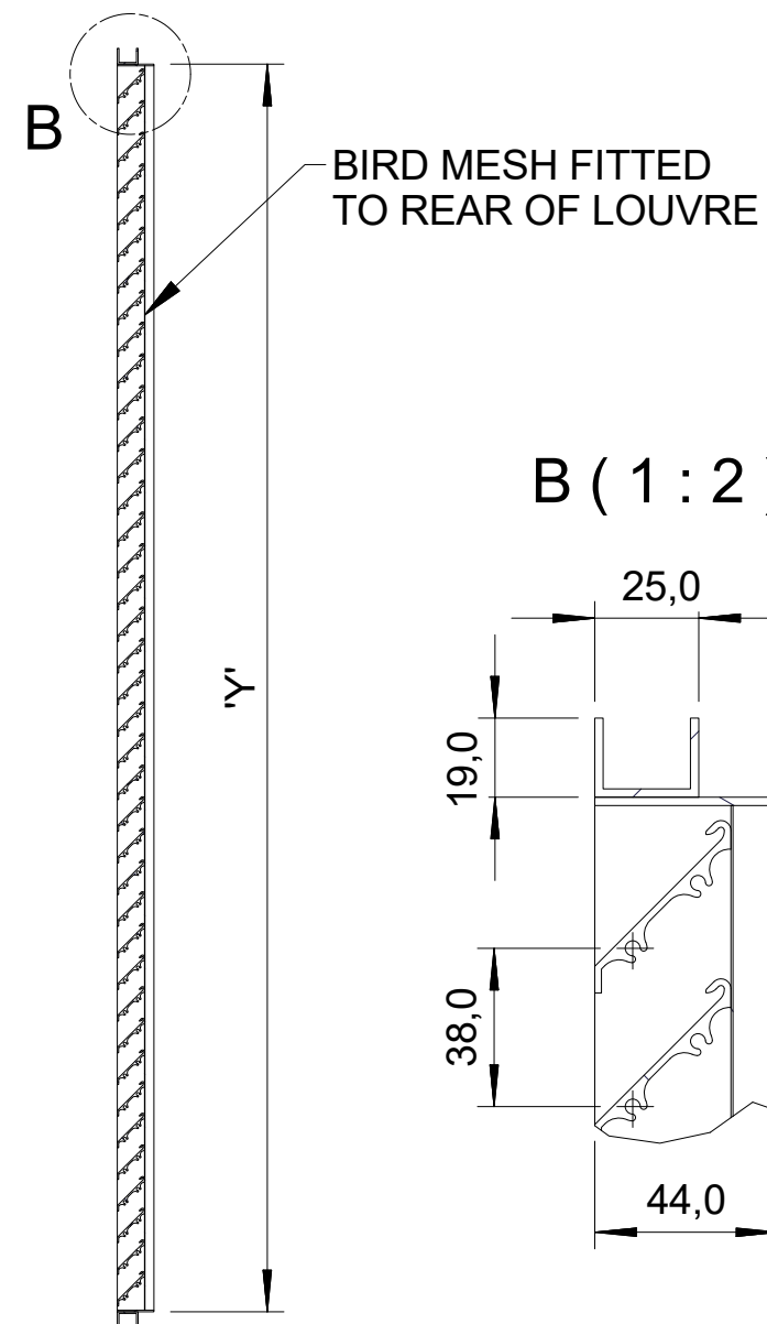
A-A ( 1 : 10 )
