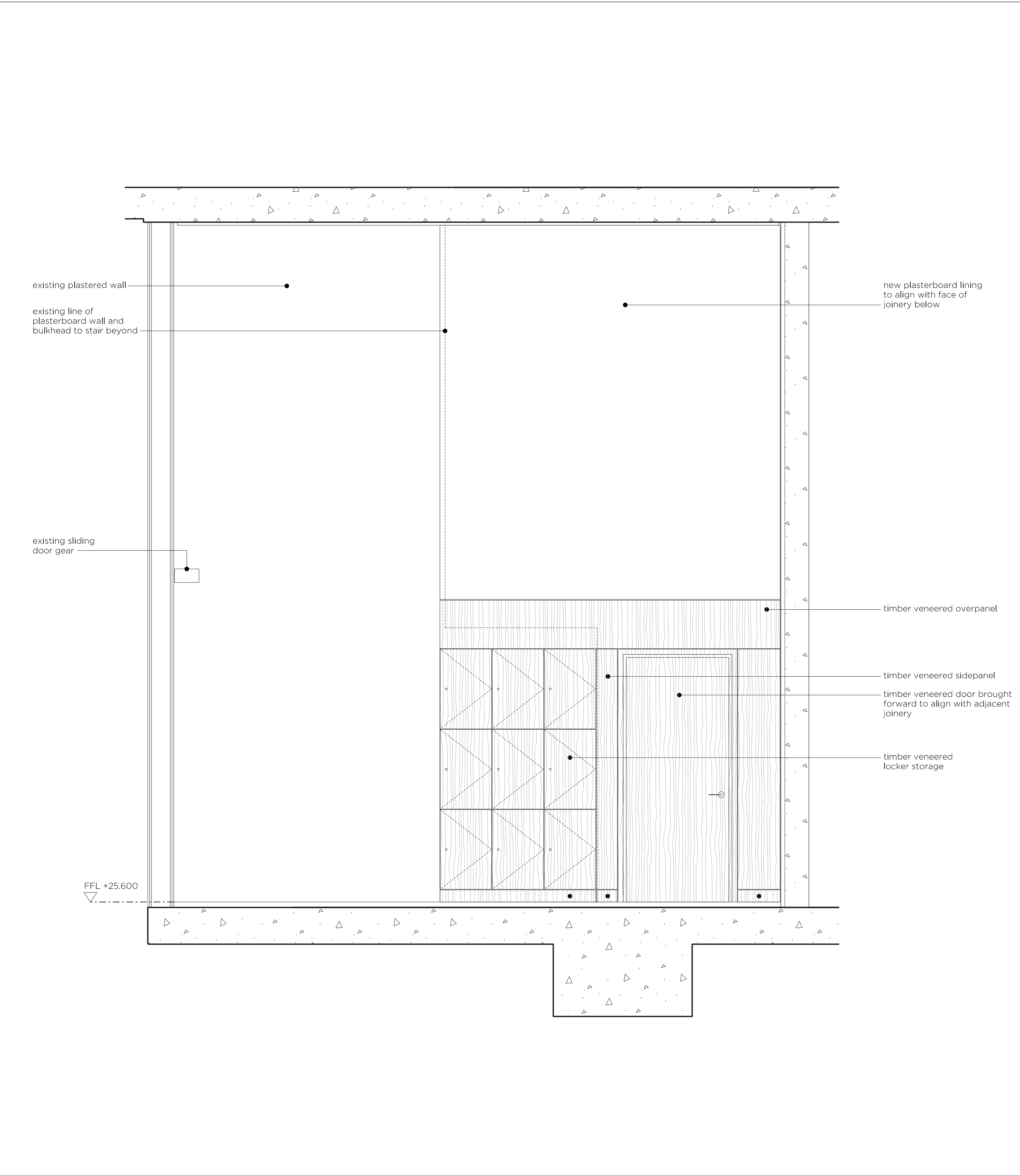
01 SECTION
