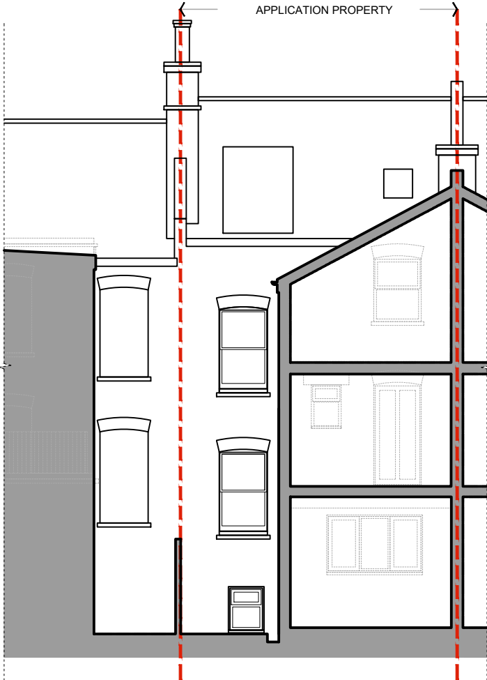
Section A-A
