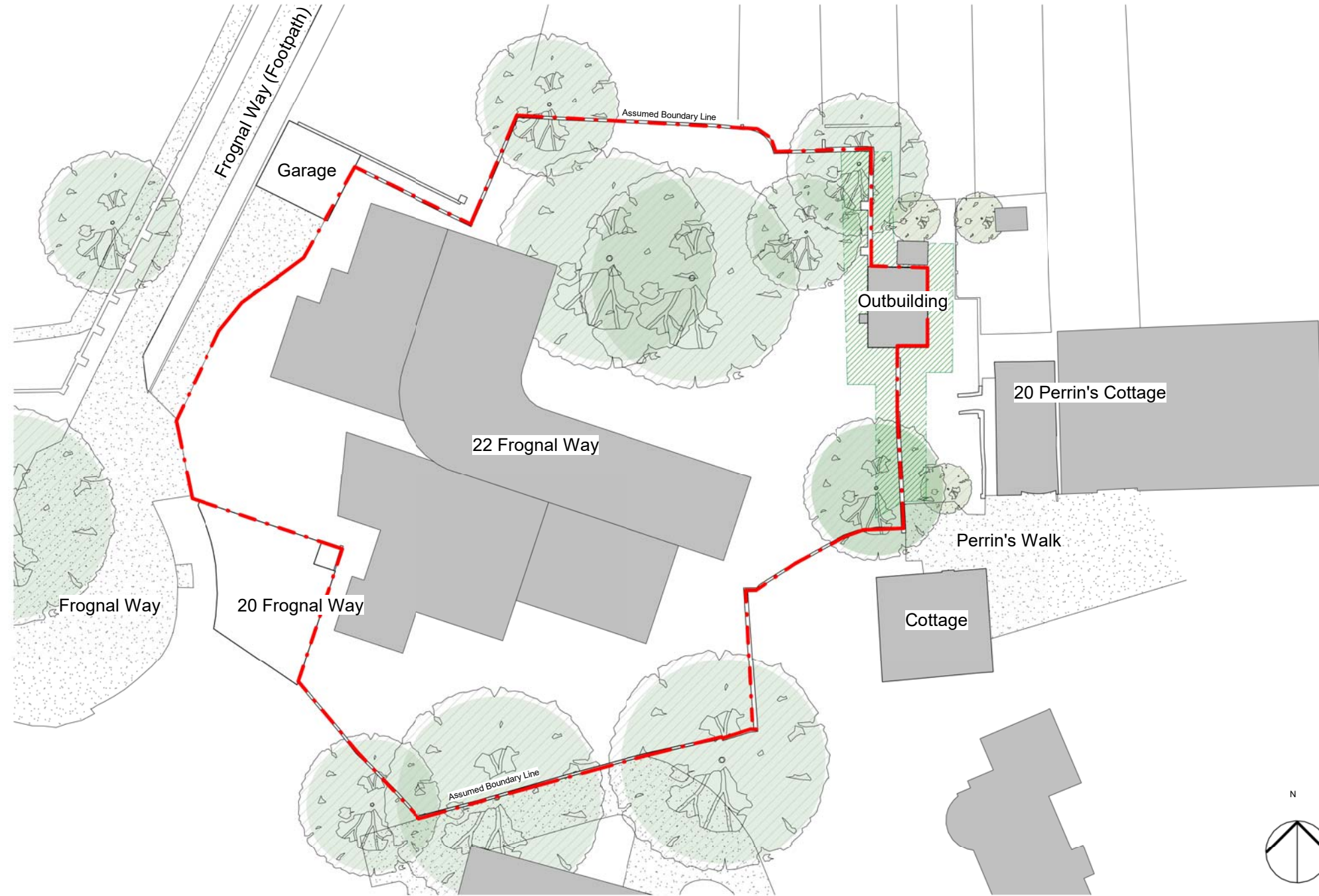
1 Site Plan 1 : 200
