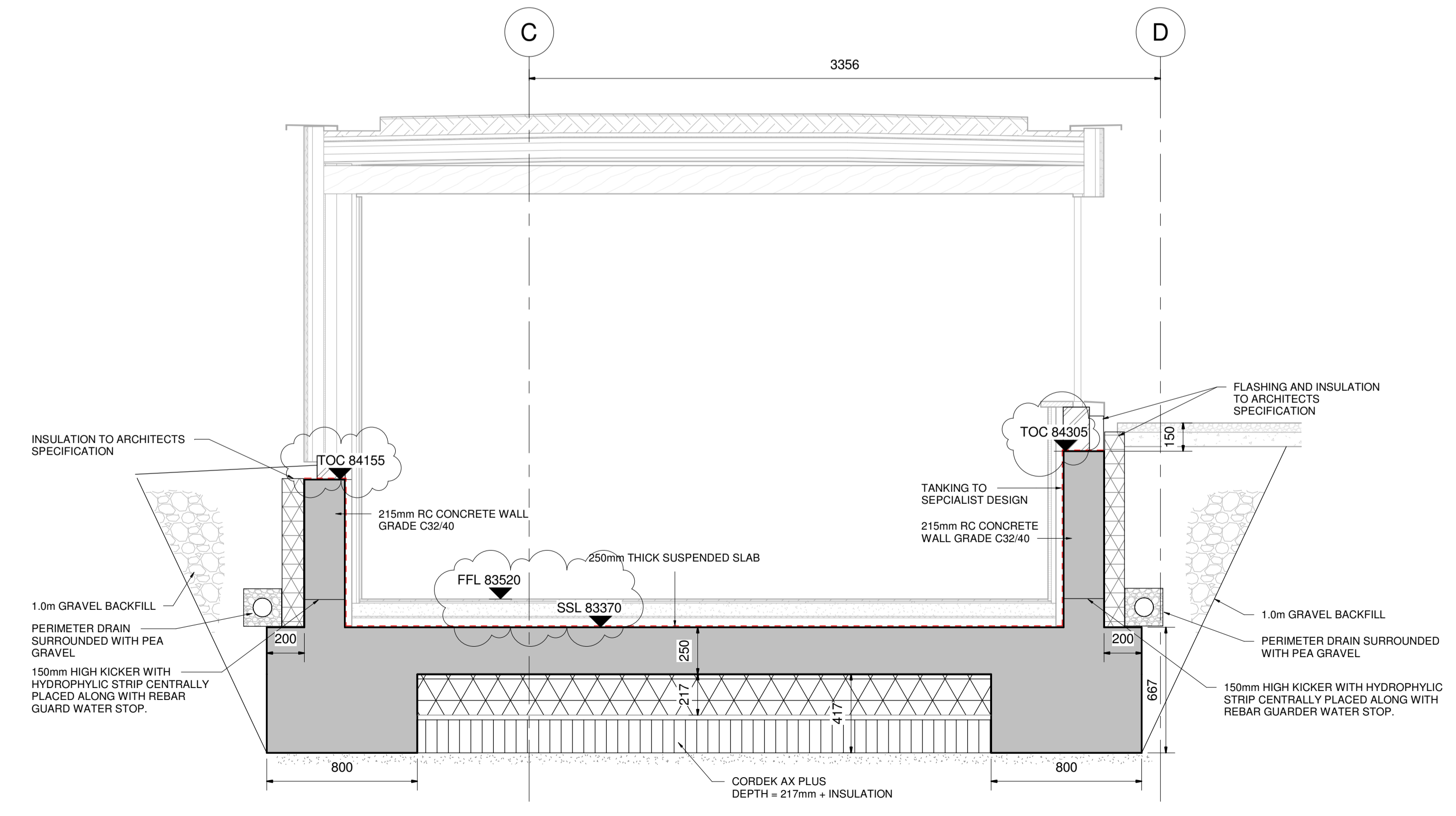
SECTION A-A 1:20
