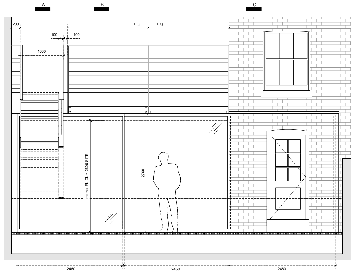
ELEVATION
