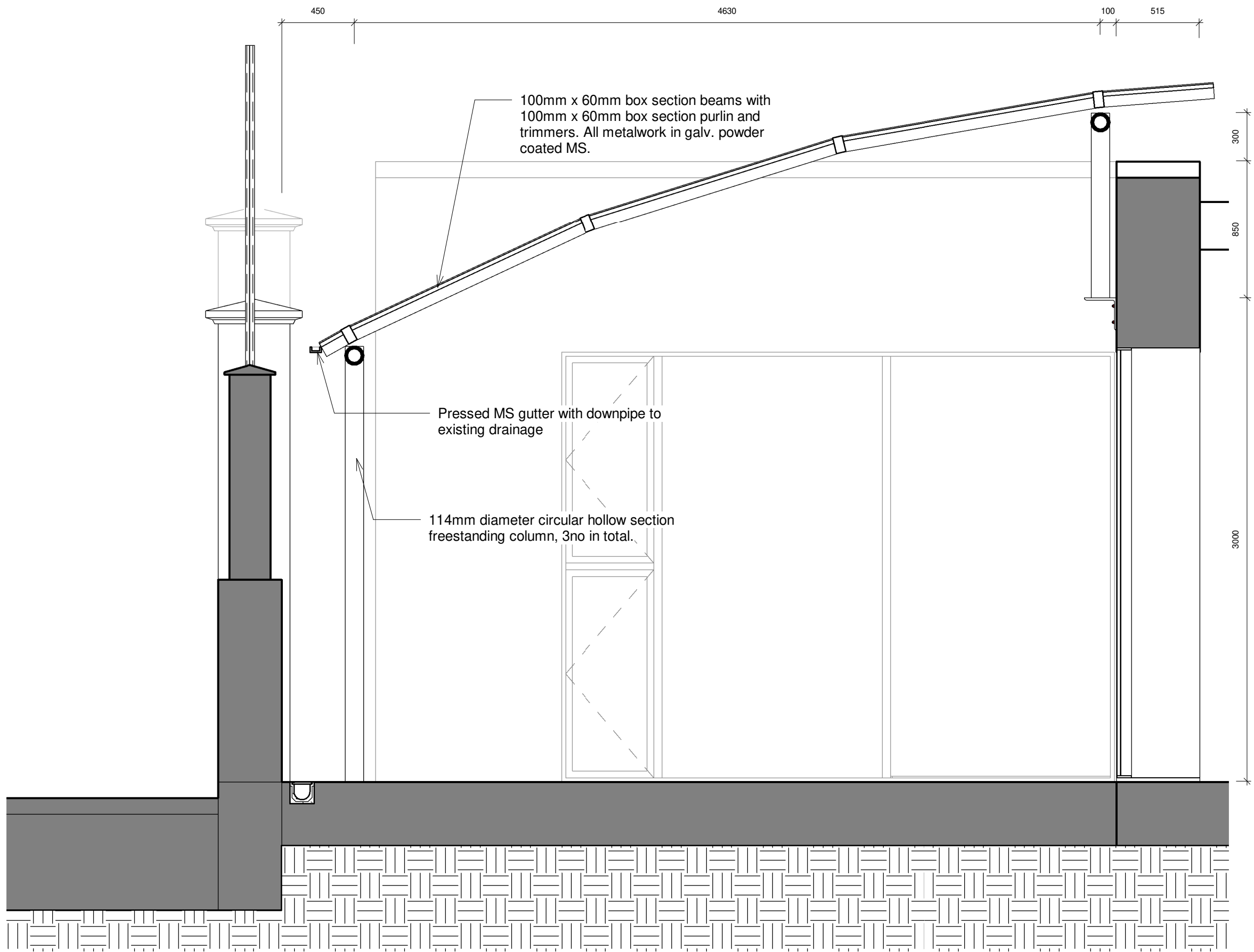
1 Cross Section 1 : 25
