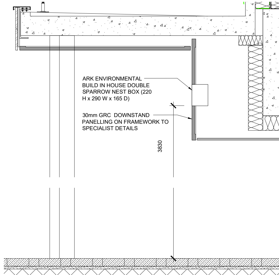
SECTION A-A 1:20
